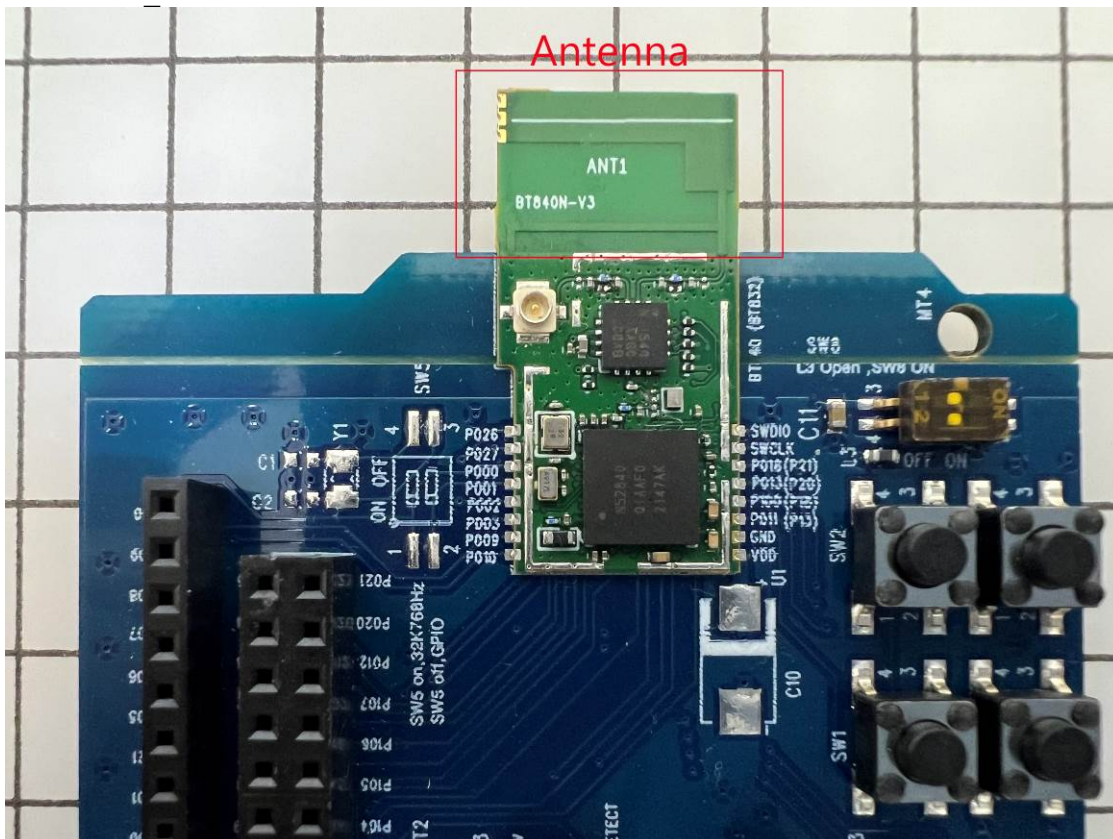
EUT-4. _Antenna
