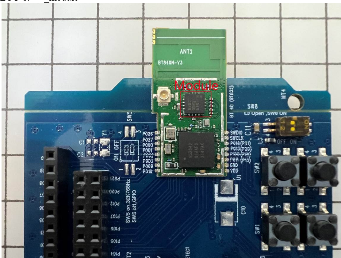
EUT-6. _module
