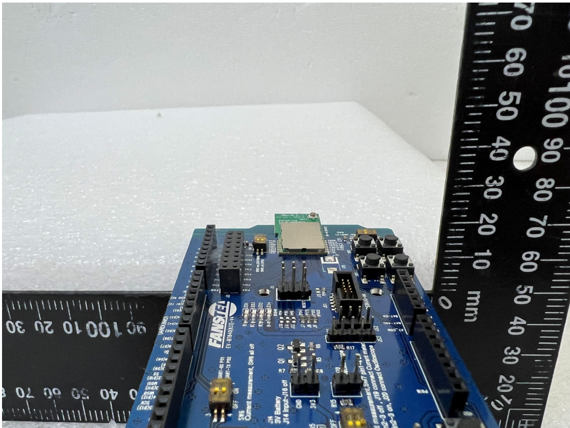
EUT-10. BT832XE
