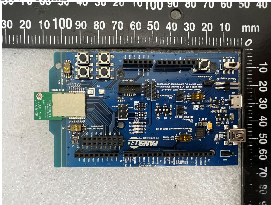
EUT-7. BT832XE
