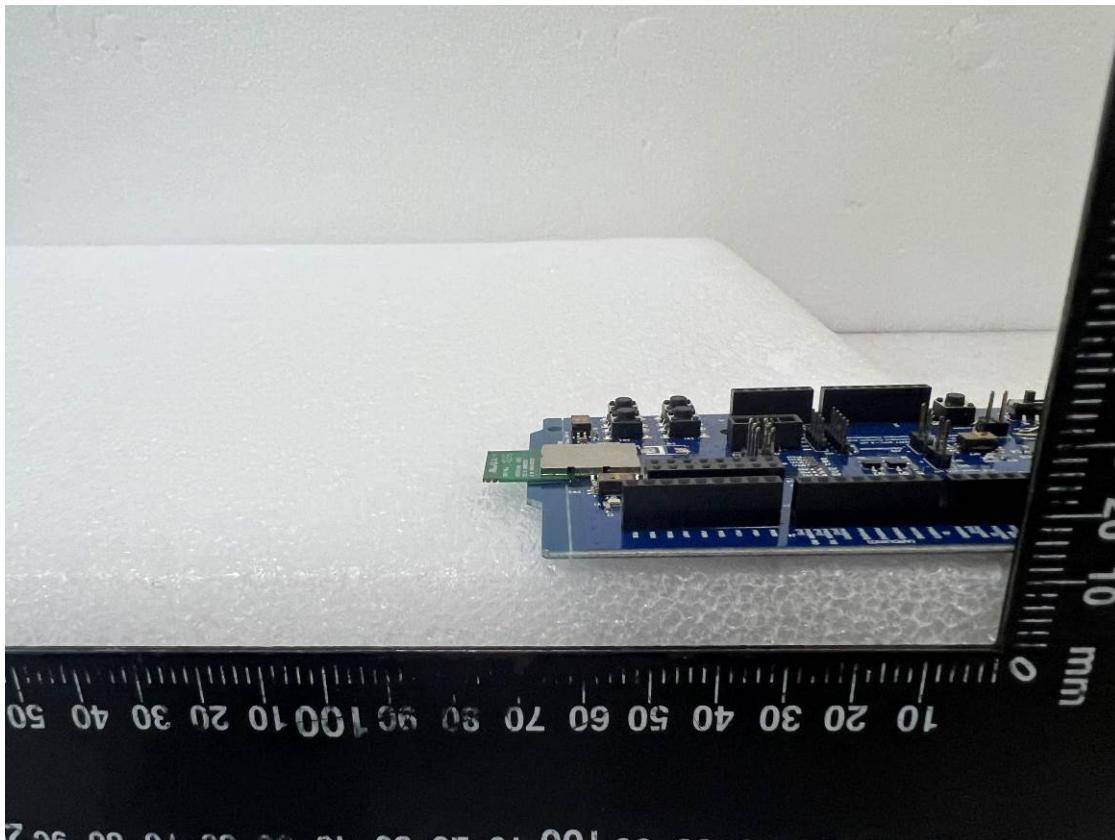
EUT-6. BT832X
