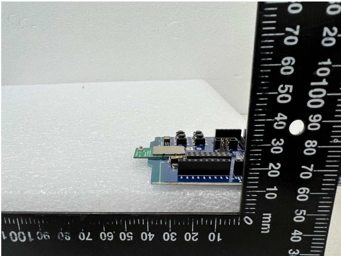
EUT-12. BT832XE
