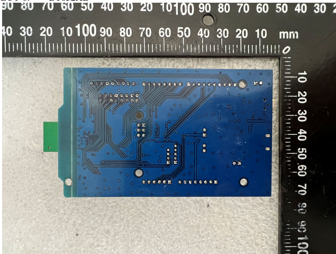
EUT-8. BT832XE
