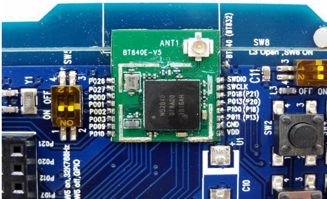
EUT 1 BT840E-1
