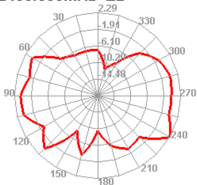
2450.000MHz E2
