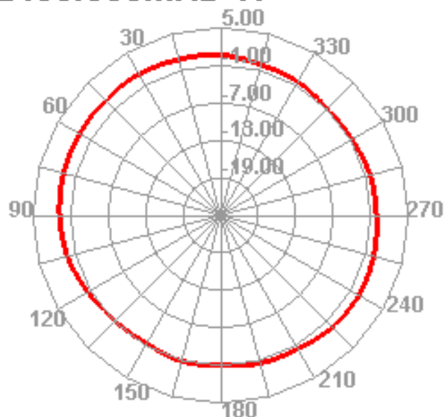
2450.000MHz H
