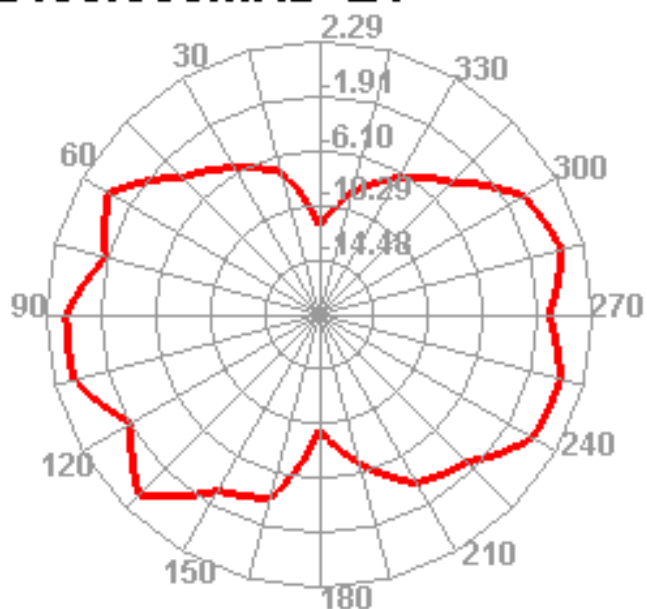
2450.000MHz E1
