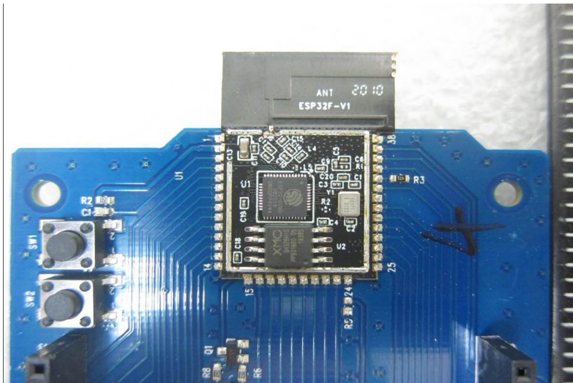
EUT 12 ESP32F
