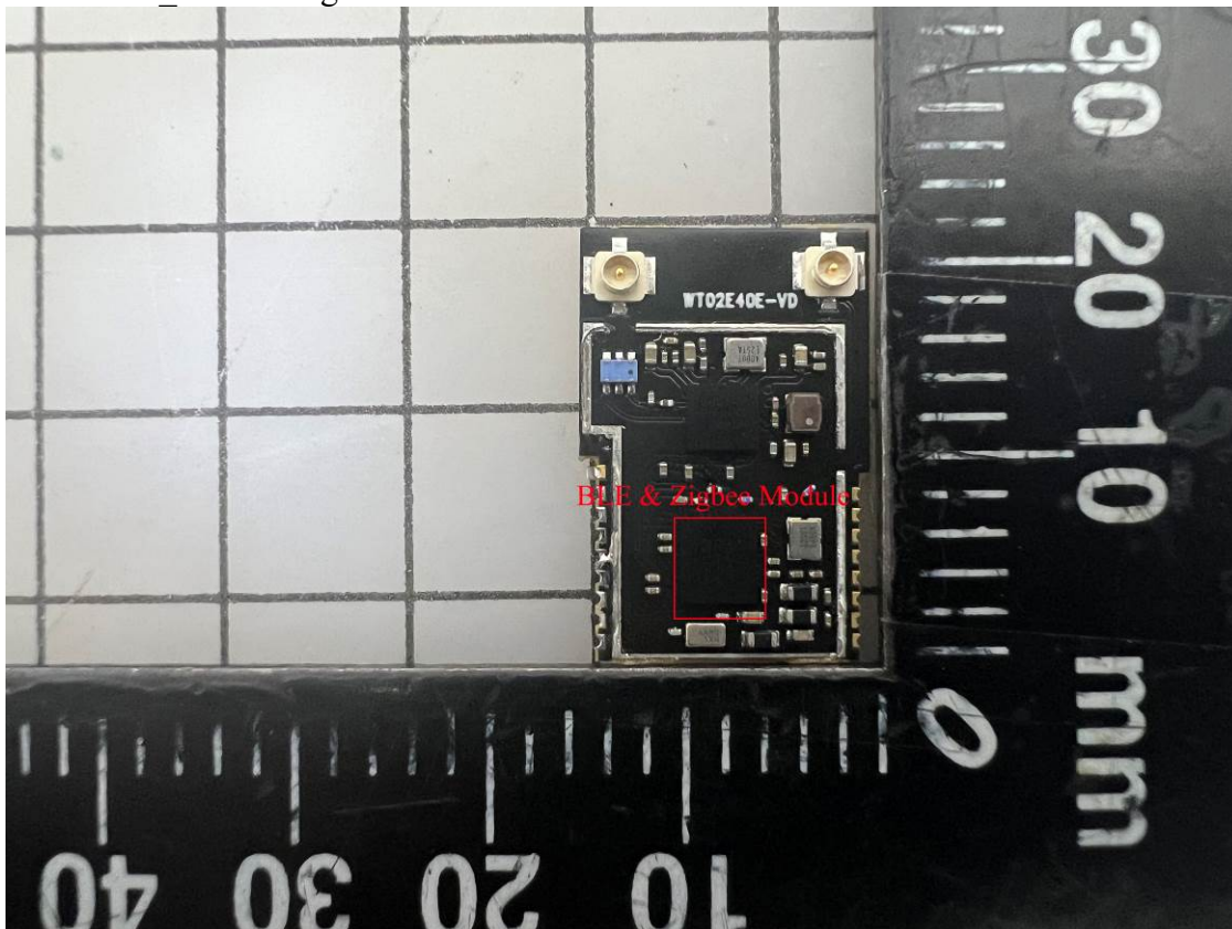
EUT-7. _BLE & Zigbee Module
