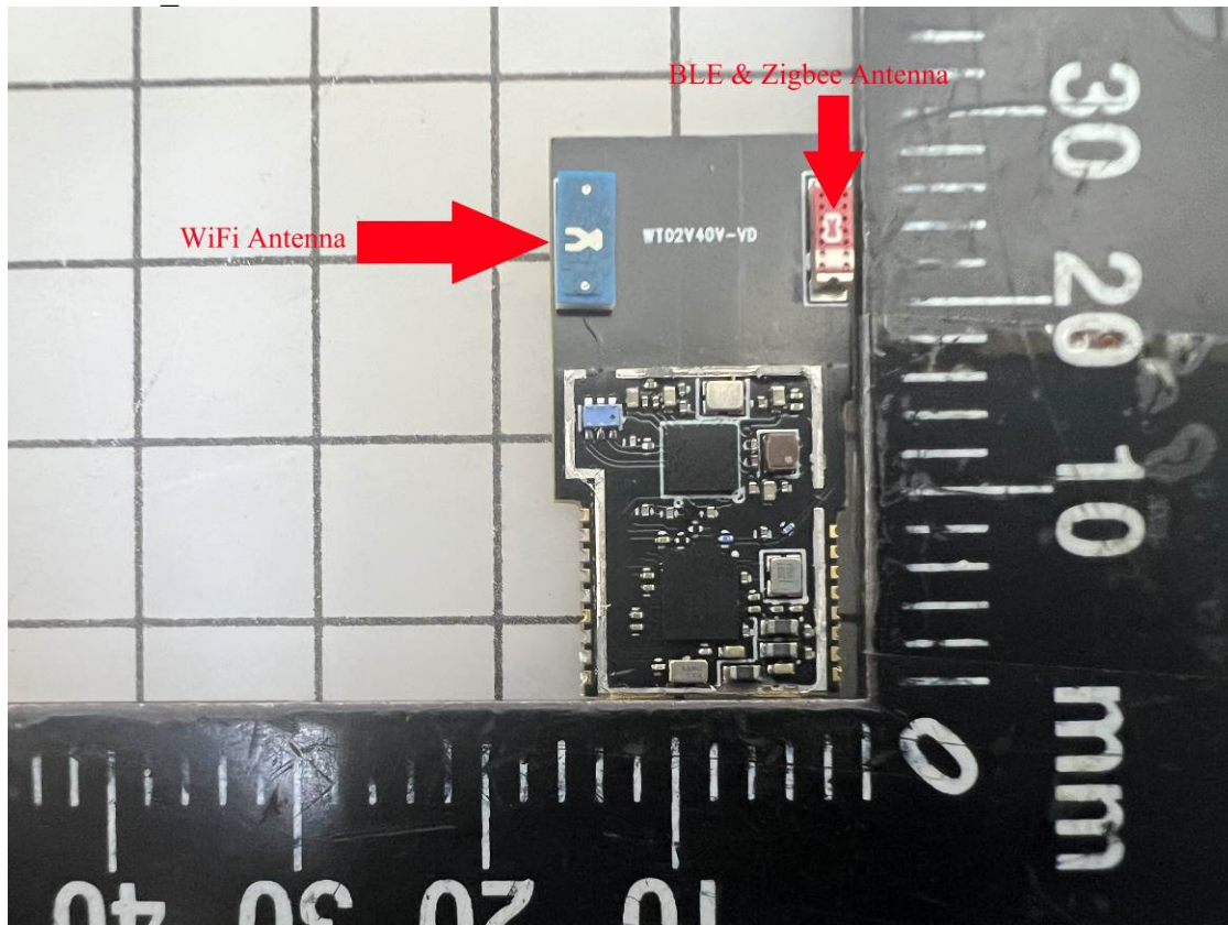
EUT-3. _WT02V40V
