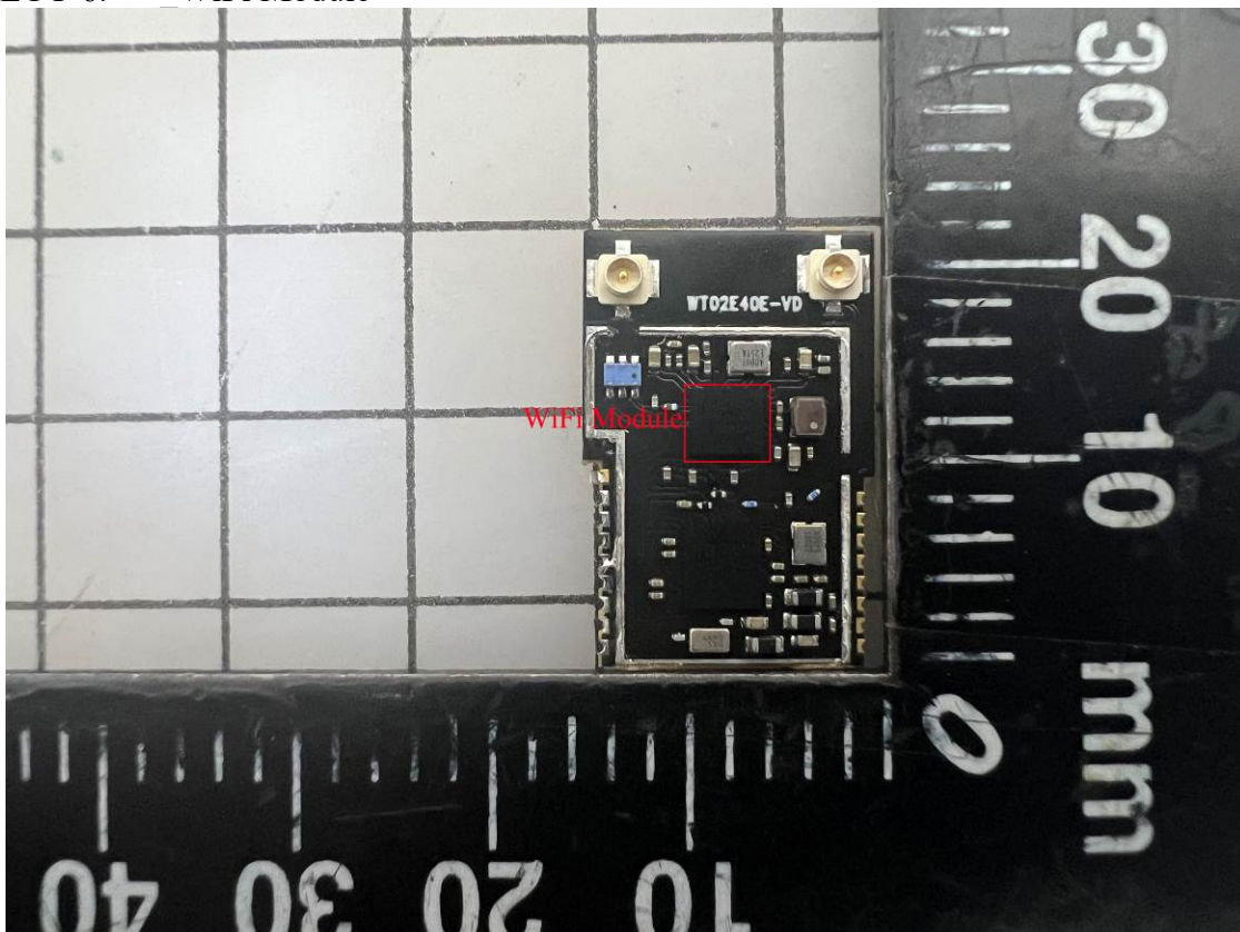
EUT-6. WiFi Module
