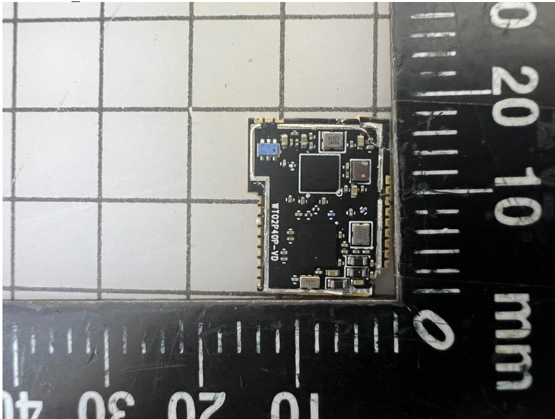
EUT-5. _WT02P40P
