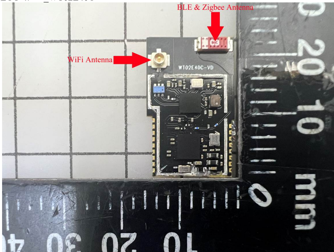
EUT-4. _WT02E40C
