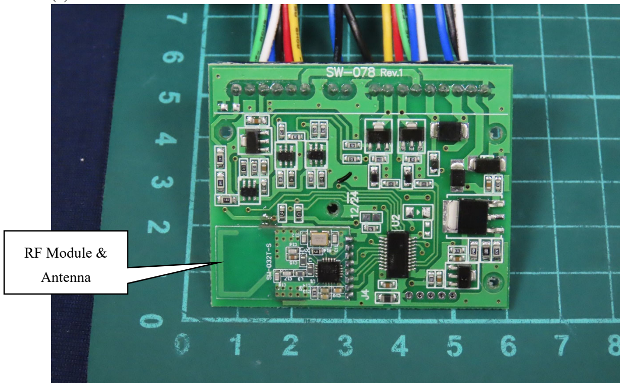
(4) EUT Photo
