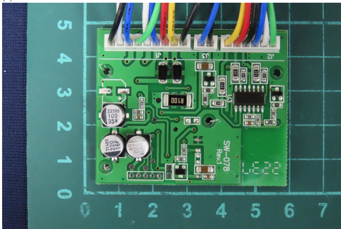
(9) EUT Photo
