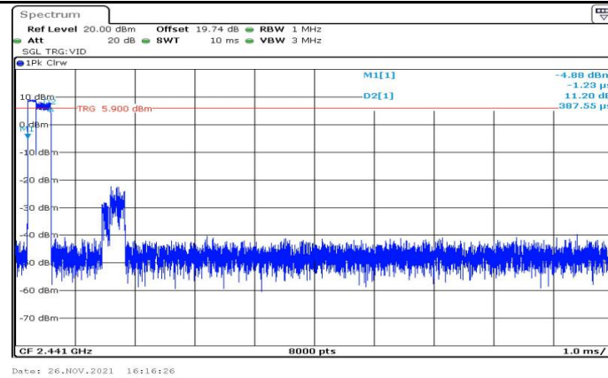
2DH1_Ant1_Hop
