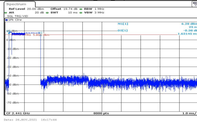
2DH3_Ant1_Hop
