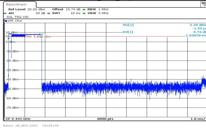
3DH3_Ant1_Hop
