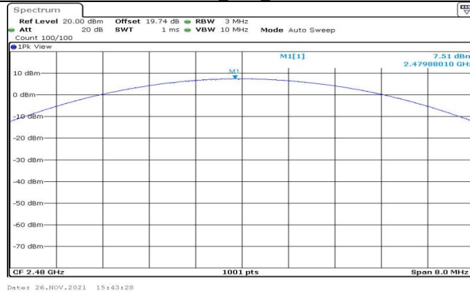
3DH1_Ant1_2480
