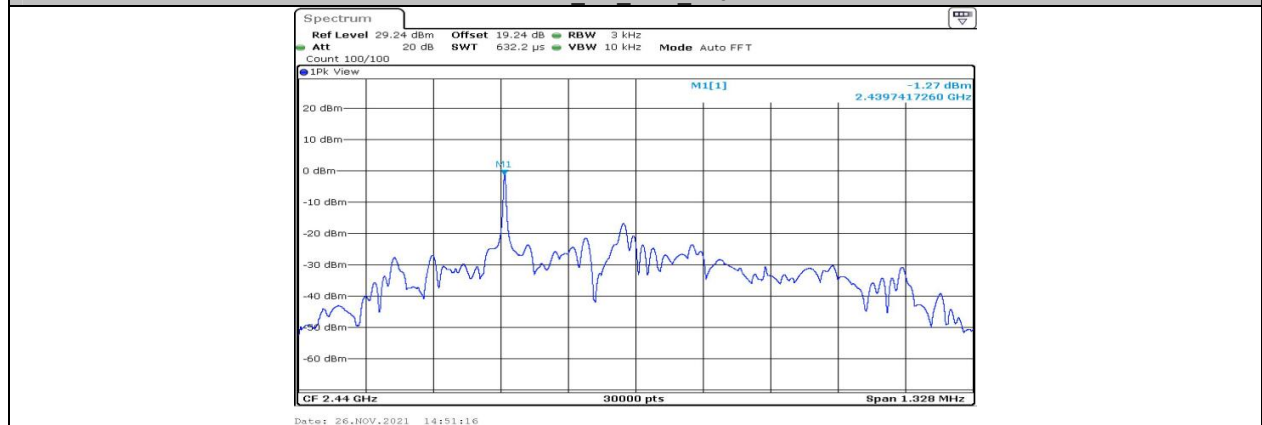
BLE_1M Ant1 2440
