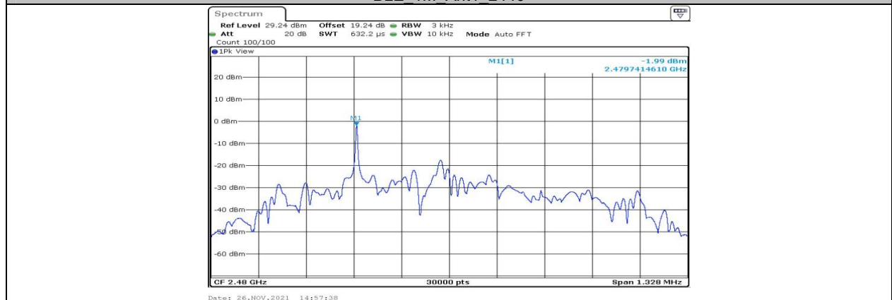
BLE_1M Ant1 2480
