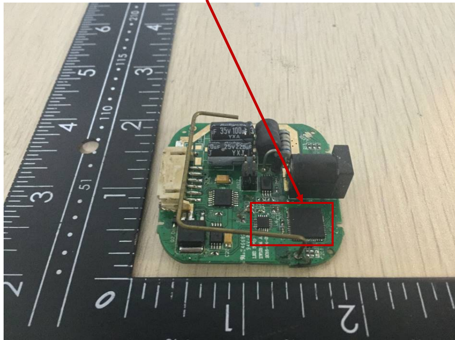
Z-WAVE Module
