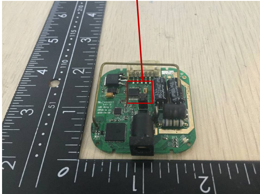
NFC Module
