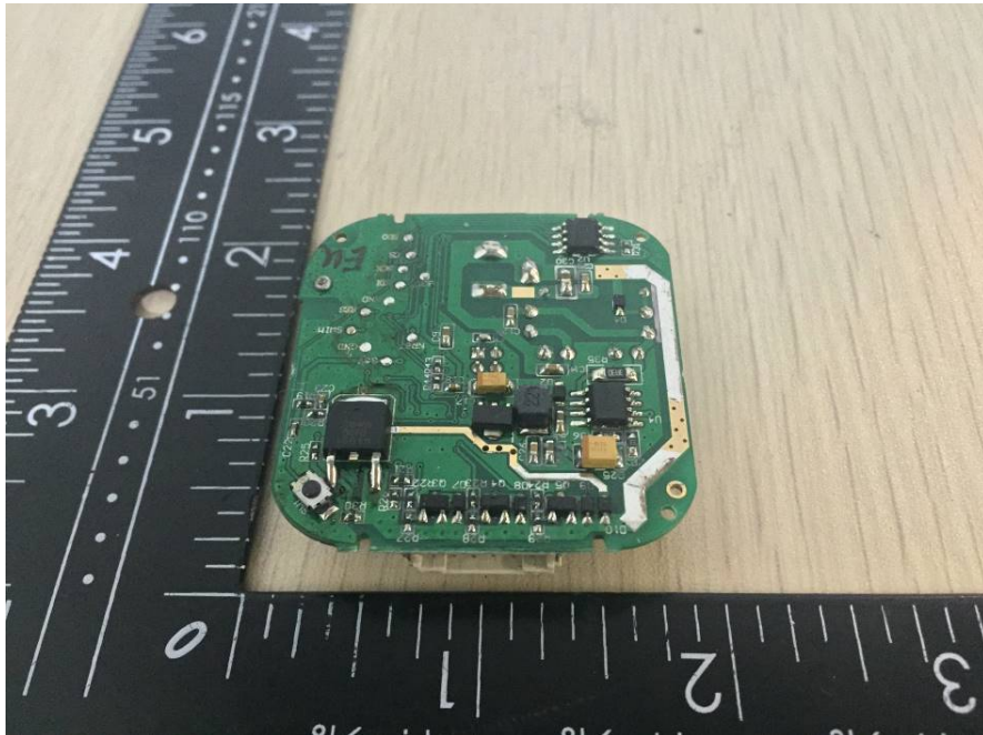
NFC Antenna
