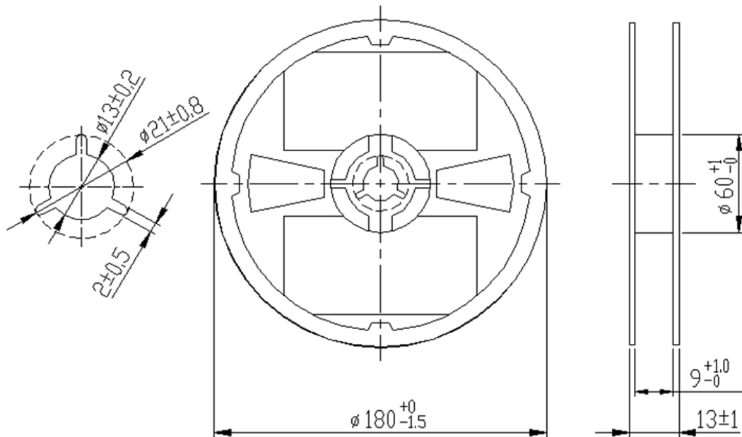
Reel Dimensions
