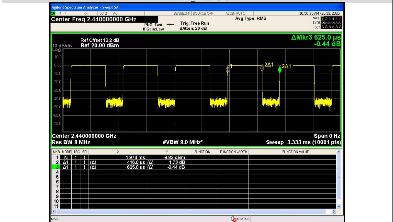
BLE 1M_Channel 19
