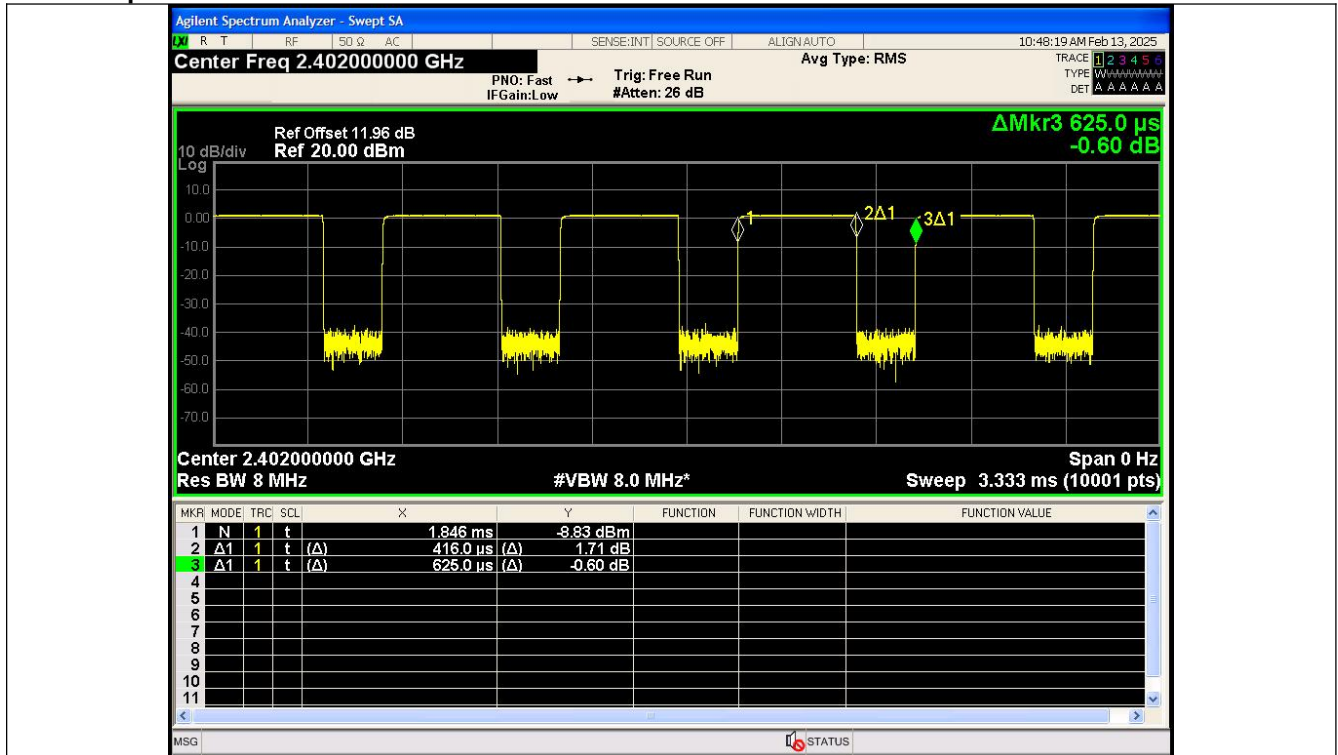
BLE 1M_Channel 0
