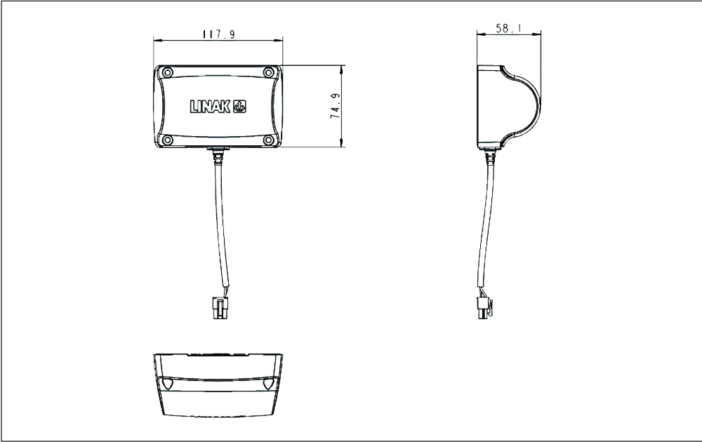
Massage motor MD1
