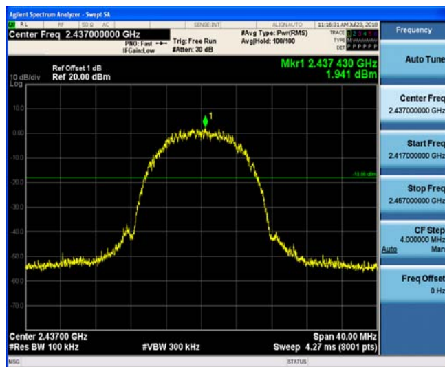
802.11b CH06
