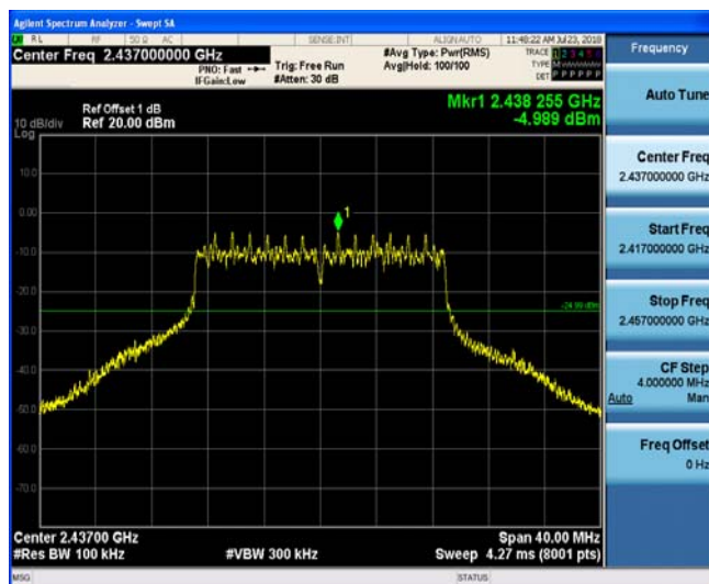
802.11n(HT20) CH06
