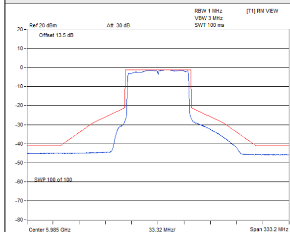
802.11ax (HE80) / Chain 0 : CH 7
