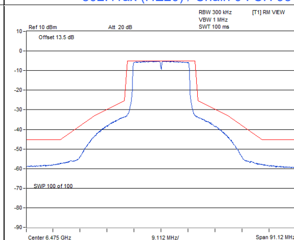
802.11ax (HE20) / Chain 0 : CH 105
