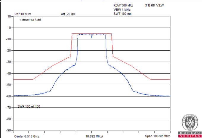
802.11ax (HE20) / Chain 3 : CH 113
