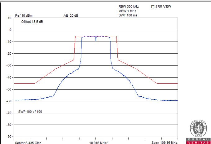
802.11ax (HE20) / Chain 3 : CH 97
