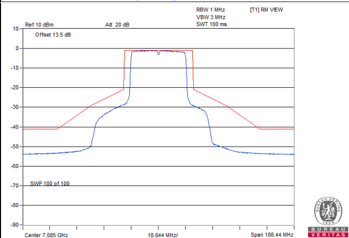
802.11ax (HE40) / Chain 1 : CH 227
