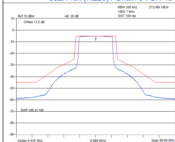
802.11ax (HE20) / Chain 0 : CH 97
