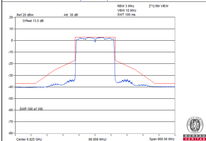
802.11ax (HE160) / Chain 3 : CH 175
