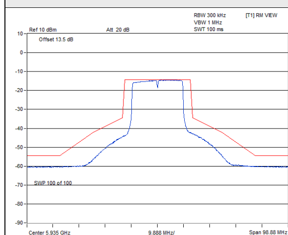
802.11ax (HE20) / Chain 0 : CH 2
