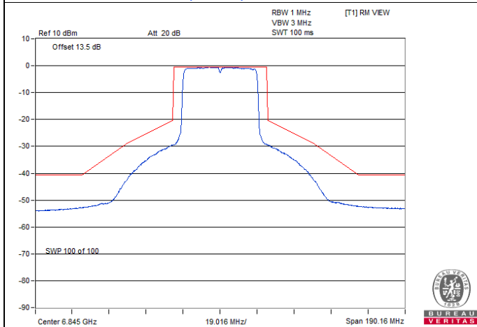
802.11ax (HE40) / Chain 2 : CH 179
