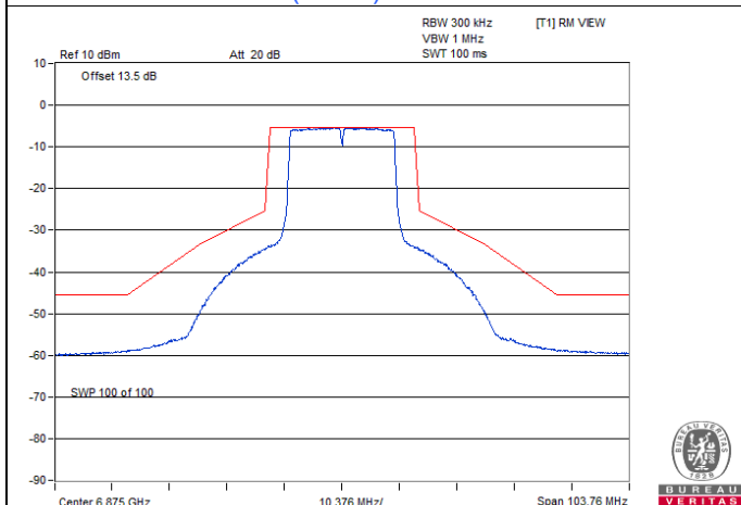
802.11ax (HE20) / Chain 0 : CH 185
