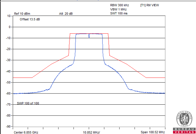
802.11ax (HE20) / Chain 0 : CH 181
