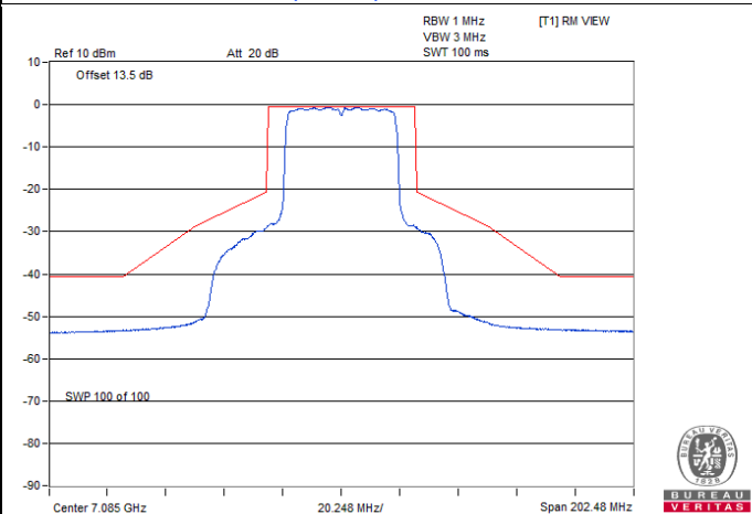
802.11ax (HE40) / Chain 2 : CH 227
