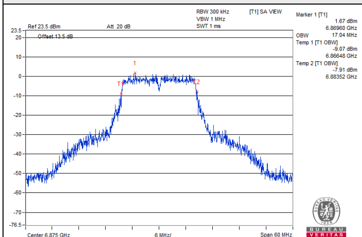
802.11a / Chain 1 : CH 185
