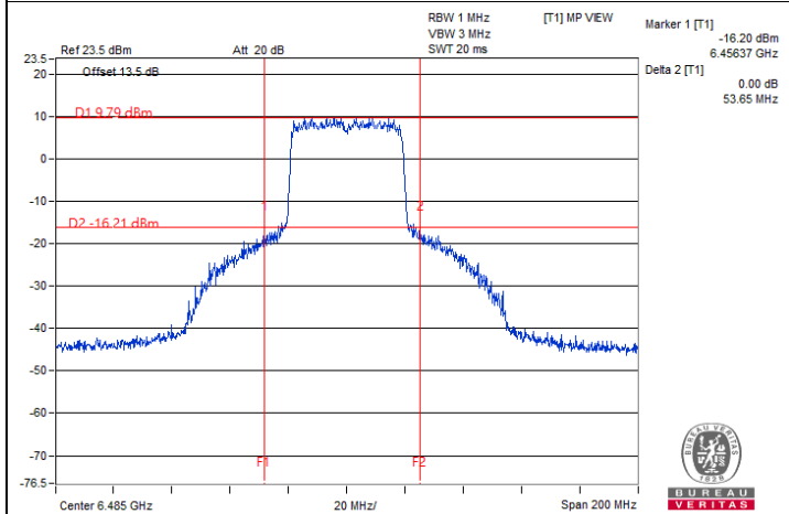
802.11ax (HE40) / Chain 1 : CH 107
