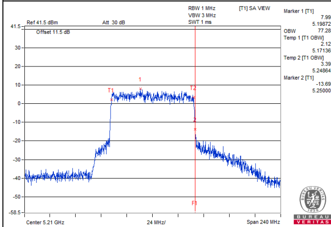
802.11ax (HE80) / Chain 2 : CH 42
