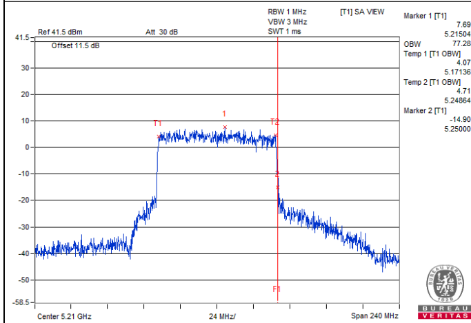
802.11ax (HE80) / Chain 0 : CH 42
