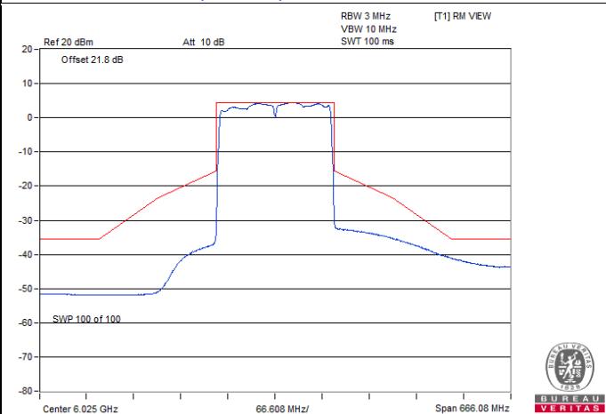
802.11ax (HE160) CDD / Chain 3 : CH 15
