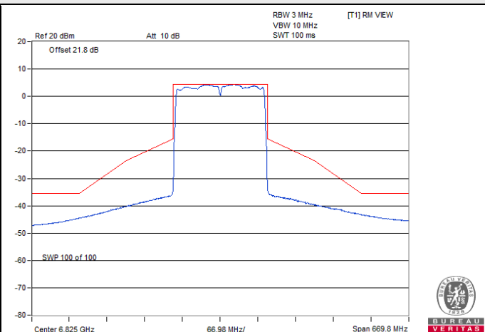
802.11ax (HE160) CDD / Chain 2 : CH 175
