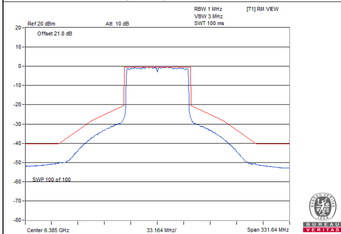
802.11ax (HE80) CDD / Chain 2 : CH 87
