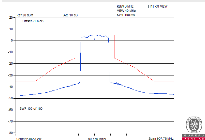
802.11ax (HE160) CDD / Chain 2 : CH 143
