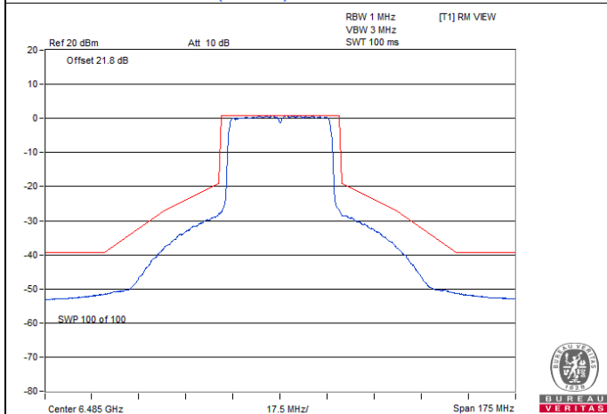
802.11ax (HE40) CDD / Chain 3 : CH 107
