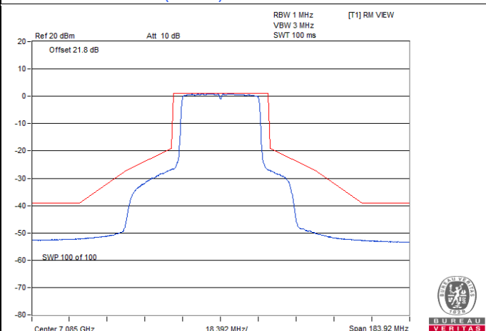
802.11ax (HE40) CDD / Chain 3 : CH 227
