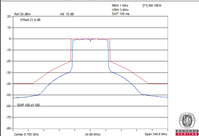
802.11ax (HE80) CDD / Chain 2 : CH 151
