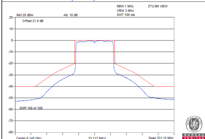
802.11ax (HE80) CDD / Chain 3 : CH 39
