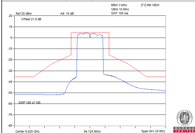
802.11ax (HE160) CDD / Chain 2 : CH 15
