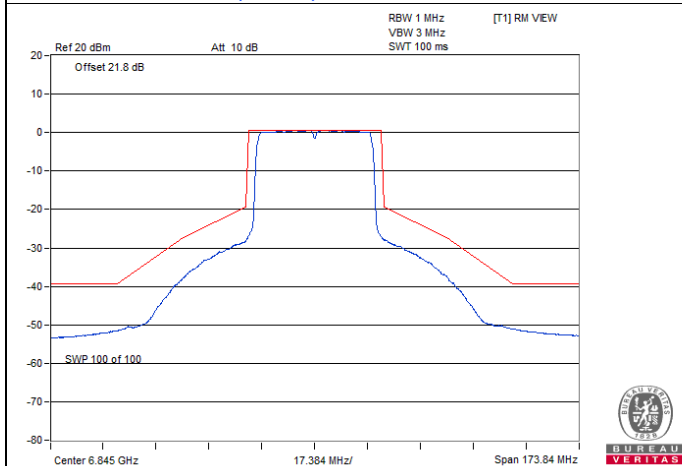
802.11ax (HE40) CDD / Chain 2 : CH 179
