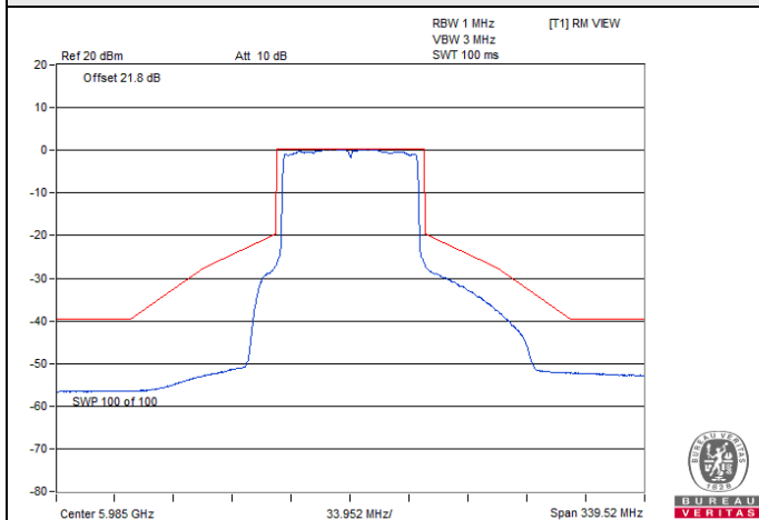
802.11ax (HE80) CDD / Chain 2 : CH 7
