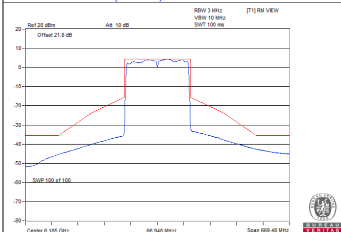
802.11ax (HE160) CDD / Chain 3 : CH 47
