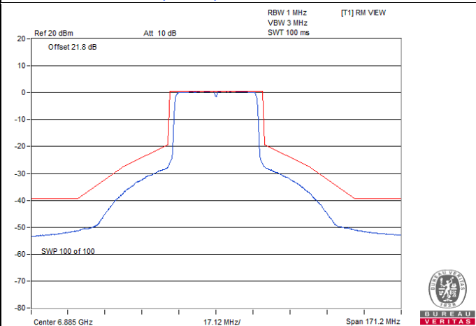
802.11ax (HE40) CDD / Chain 2 : CH 187
