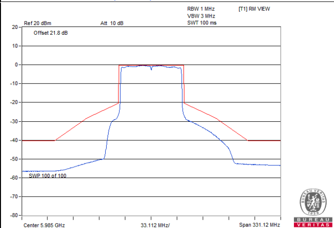
802.11ax (HE80) CDD / Chain 1 : CH 7
