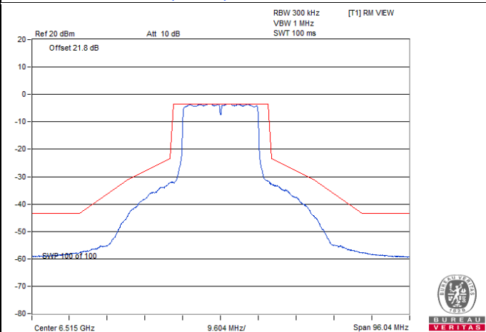
802.11ax (HE20) CDD / Chain 3 : CH 113
