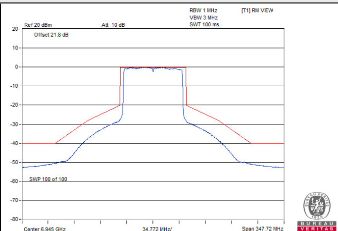
802.11ax (HE80) CDD / Chain 0 : CH 199
