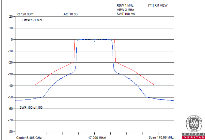
802.11ax (HE40) CDD / Chain 3 : CH 91
