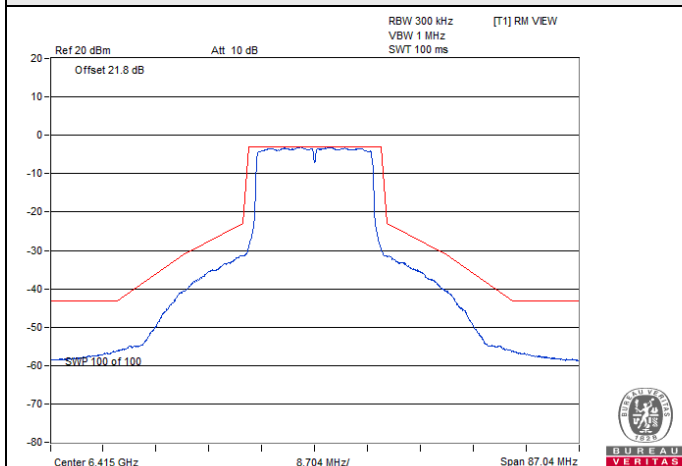
802.11ax (HE20) CDD / Chain 3 : CH 93
