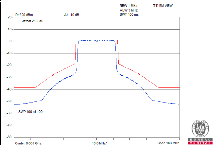
802.11ax (HE40) CDD / Chain 3 : CH 187
