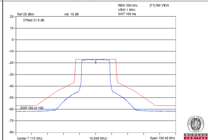
802.11ax (HE20) CDD / Chain 3 : CH 233
