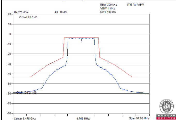
802.11ax (HE20) CDD / Chain 3 : CH 105
