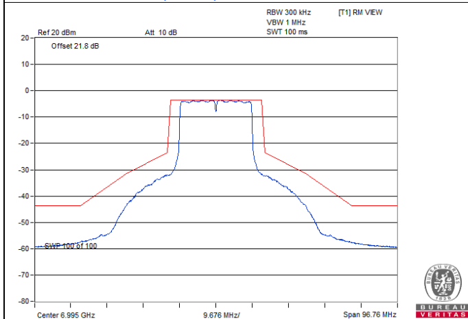
802.11ax (HE20) CDD / Chain 3 : CH 209
