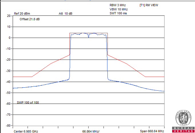
802.11ax (HE160) CDD / Chain 3 : CH 207
