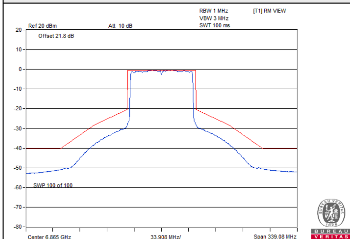
802.11ax (HE80) CDD / Chain 2 : CH 183
