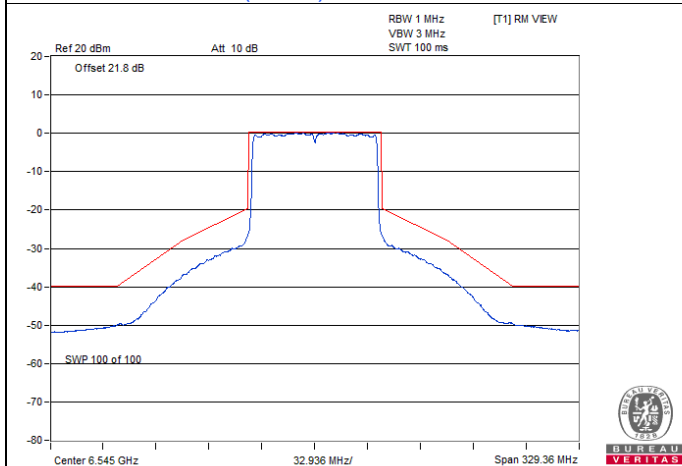
802.11ax (HE80) CDD / Chain 2 : CH 119
