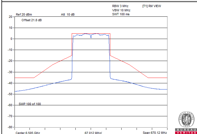
802.11ax (HE160) CDD / Chain 3 : CH 111
