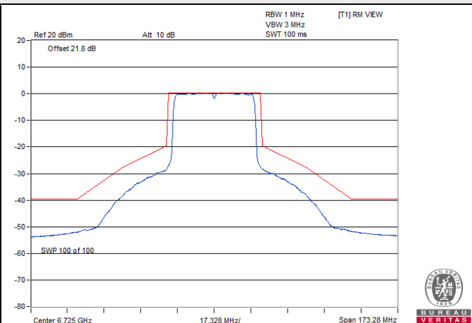
802.11ax (HE40) CDD / Chain 2 : CH 155
