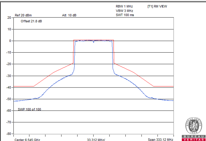
802.11ax (HE80) CDD / Chain 3 : CH 119
