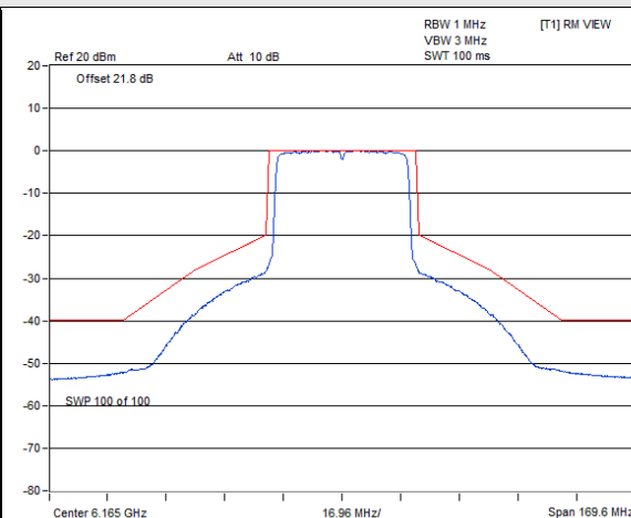
802.11ax (HE40) CDD / Chain 0 : CH 43
