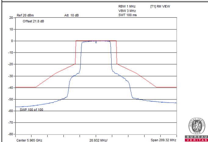
802.11ax (HE40) CDD / Chain 3 : CH 3
