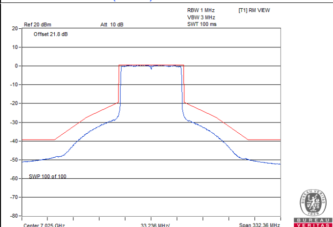
802.11ax (HE80) CDD / Chain 3 : CH 215
