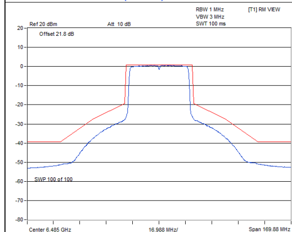
802.11ax (HE40) CDD / Chain 0 : CH 107
