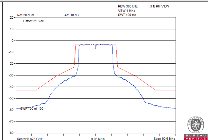
802.11ax (HE20) CDD / Chain 3 : CH 185
