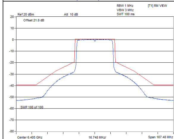
802.11ax (HE40) CDD / Chain 0 : CH 91
