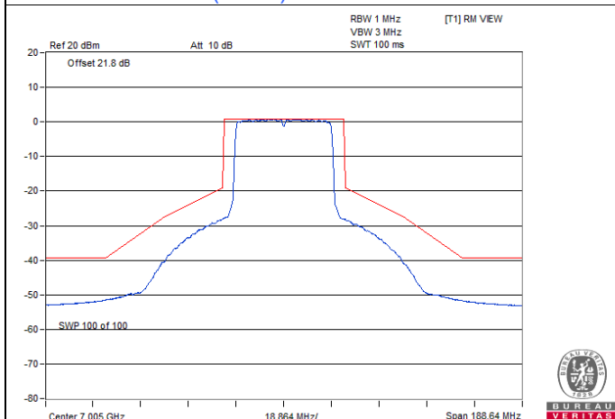
802.11ax (HE40) CDD / Chain 3 : CH 211
