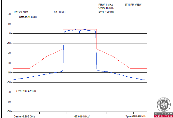
802.11ax (HE160) CDD / Chain 2 : CH 207
