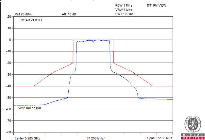
802.11ax (HE80) CDD / Chain 3 : CH 7
