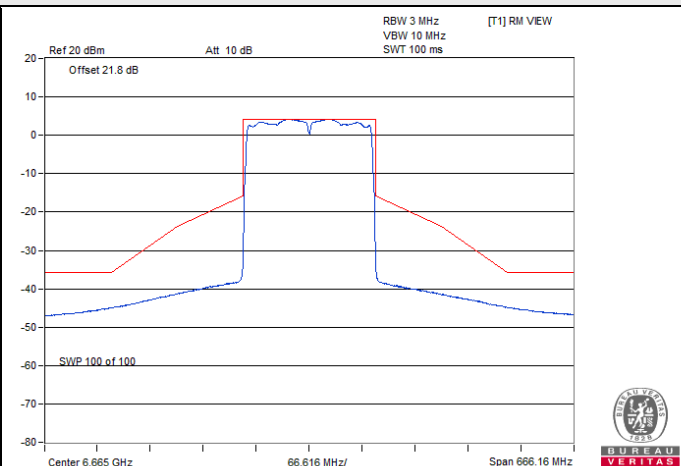
802.11ax (HE160) CDD / Chain 3 : CH 143
