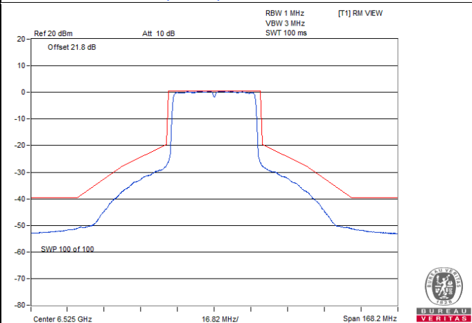
802.11ax (HE40) CDD / Chain 2 : CH 115
