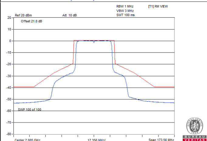
802.11ax (HE40) CDD / Chain 2 : CH 227
