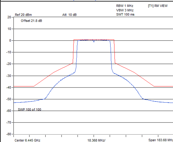
802.11ax (HE40) CDD / Chain 0 : CH 99
