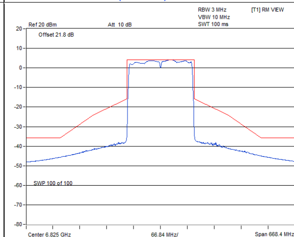
802.11ax (HE160) CDD / Chain 0 : CH 175
