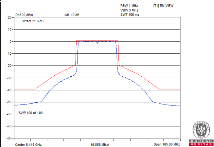
802.11ax (HE40) CDD / Chain 2 : CH 99
