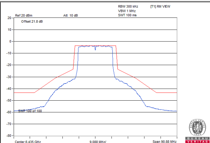
802.11ax (HE20) CDD / Chain 3 : CH 97
