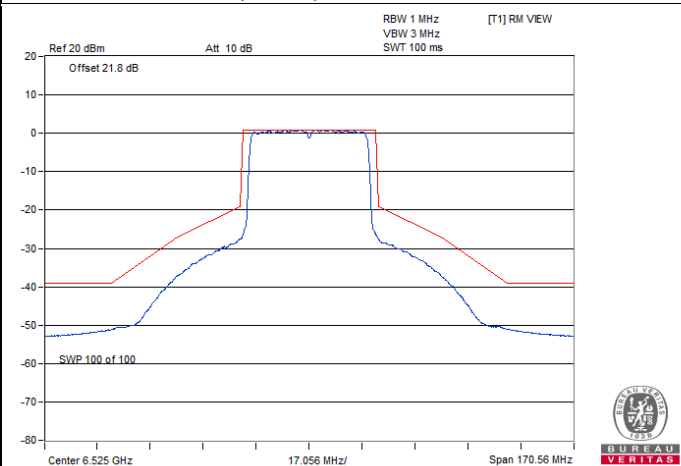
802.11ax (HE40) CDD / Chain 3 : CH 115
