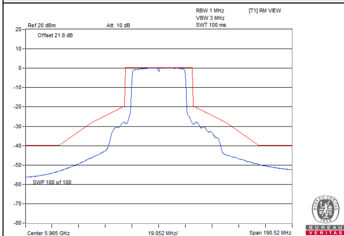
802.11ax (HE40) CDD / Chain 2 : CH 3
