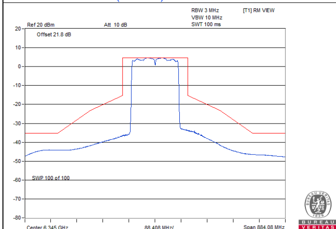
802.11ax (HE160) CDD / Chain 2 : CH 79
