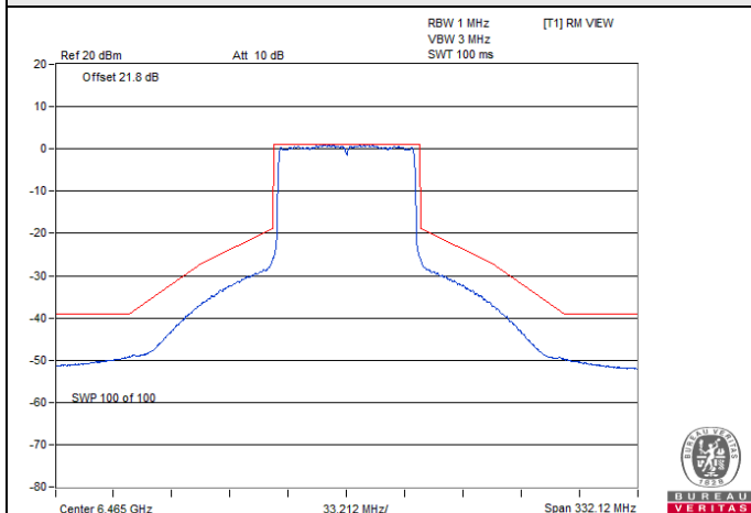
802.11ax (HE80) CDD / Chain 3 : CH 103
