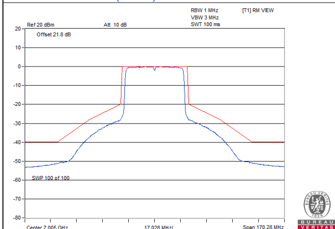
802.11ax (HE40) CDD / Chain 2 : CH 211
