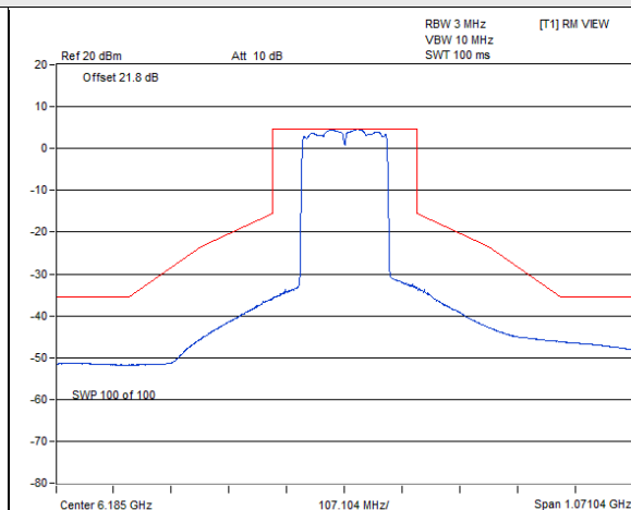
802.11ax (HE160) CDD / Chain 0 : CH 47
