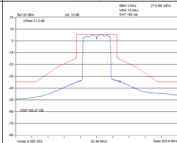
802.11ax (HE160) CDD / Chain 0 : CH 111
