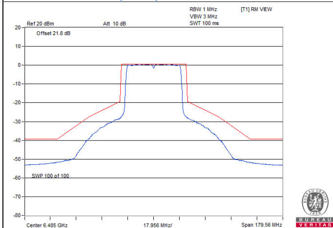
802.11ax (HE40) CDD / Chain 2 : CH 107
