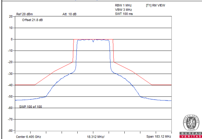
802.11ax (HE40) CDD / Chain 2 : CH 91
