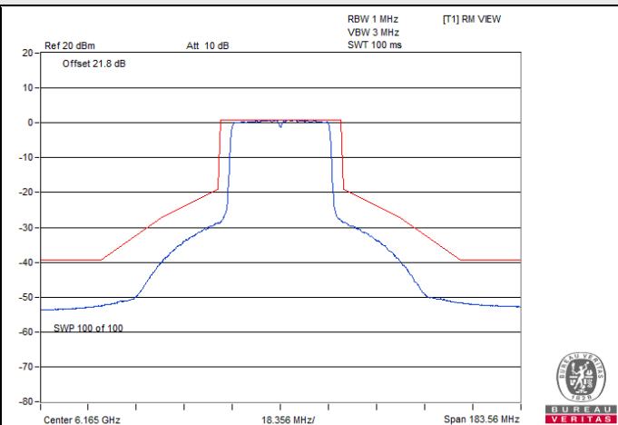
802.11ax (HE40) CDD / Chain 3 : CH 43
