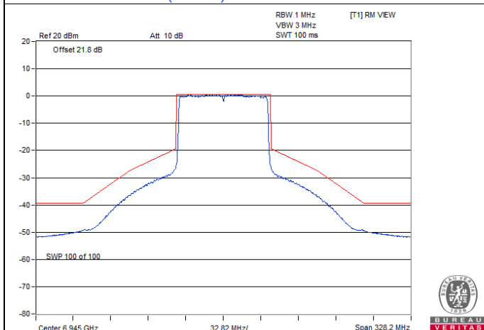
802.11ax (HE80) CDD / Chain 3 : CH 199
