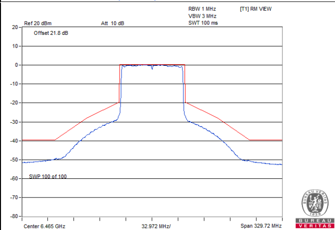
802.11ax (HE80) CDD / Chain 2 : CH 103
