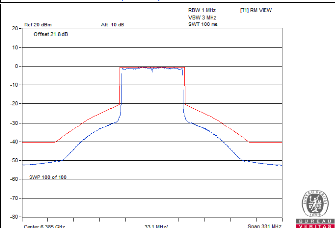
802.11ax (HE80) CDD / Chain 3 : CH 87
