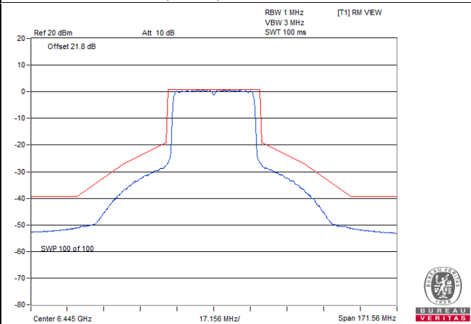
802.11ax (HE40) CDD / Chain 3 : CH 99
