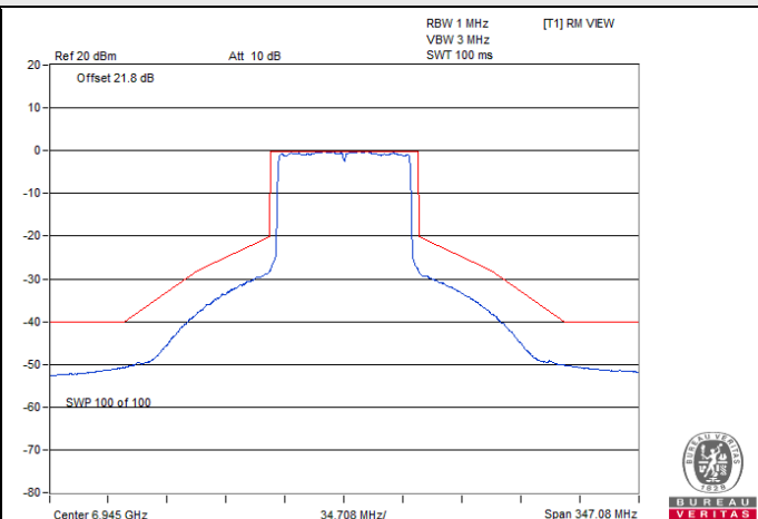
802.11ax (HE80) CDD / Chain 2 : CH 199
