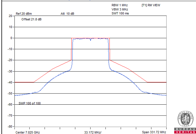
802.11ax (HE80) CDD / Chain 2 : CH 215
