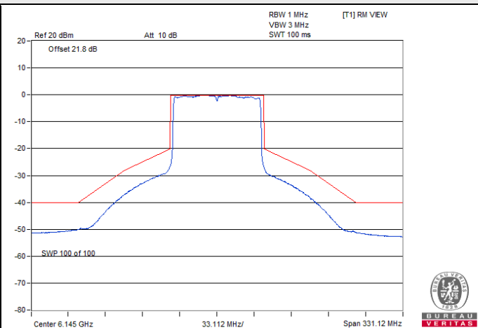
802.11ax (HE80) CDD / Chain 2 : CH 39
