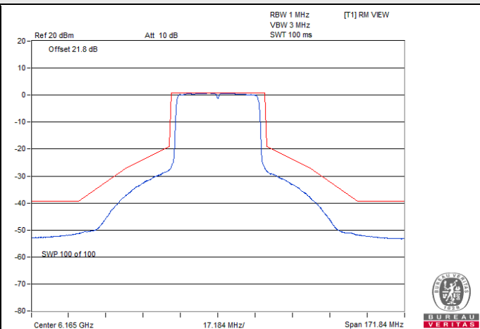
802.11ax (HE40) CDD / Chain 2 : CH 43
