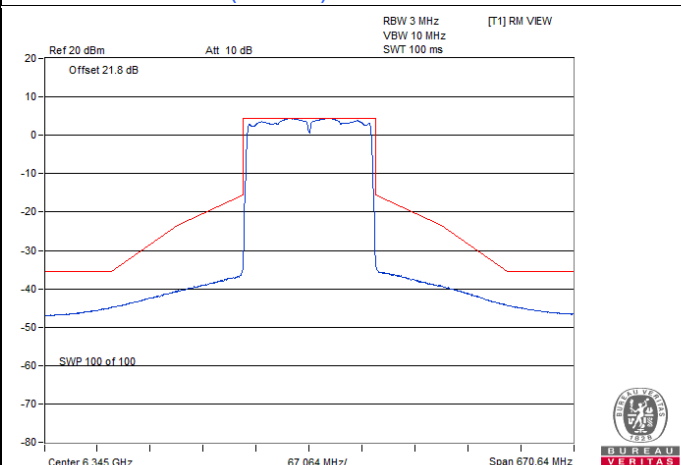
802.11ax (HE160) CDD / Chain 3 : CH 79
