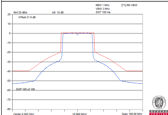
802.11ax (HE40) CDD / Chain 2 : CH 123
