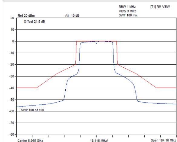
802.11ax (HE40) CDD / Chain 0 : CH 3
