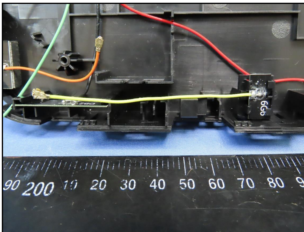
6G6 antenna
