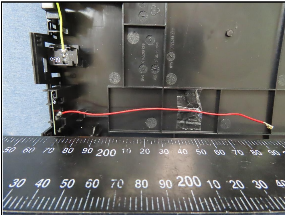
6G5 antenna
