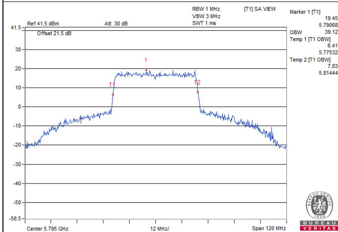
802.11ax (HE40) / Chain 2 : CH 159
