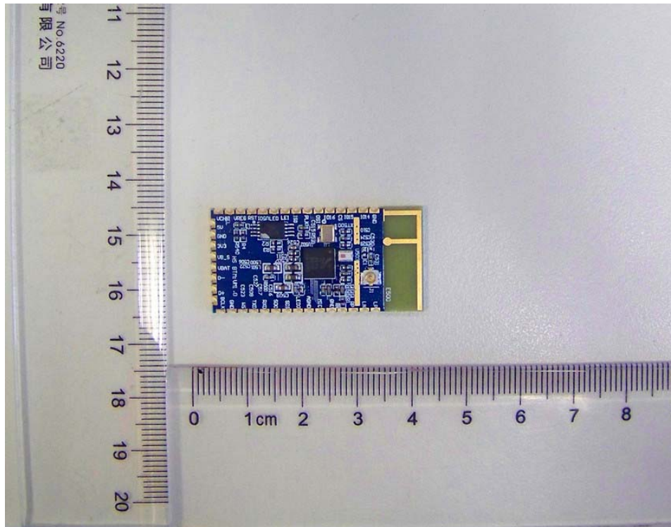
BT module
