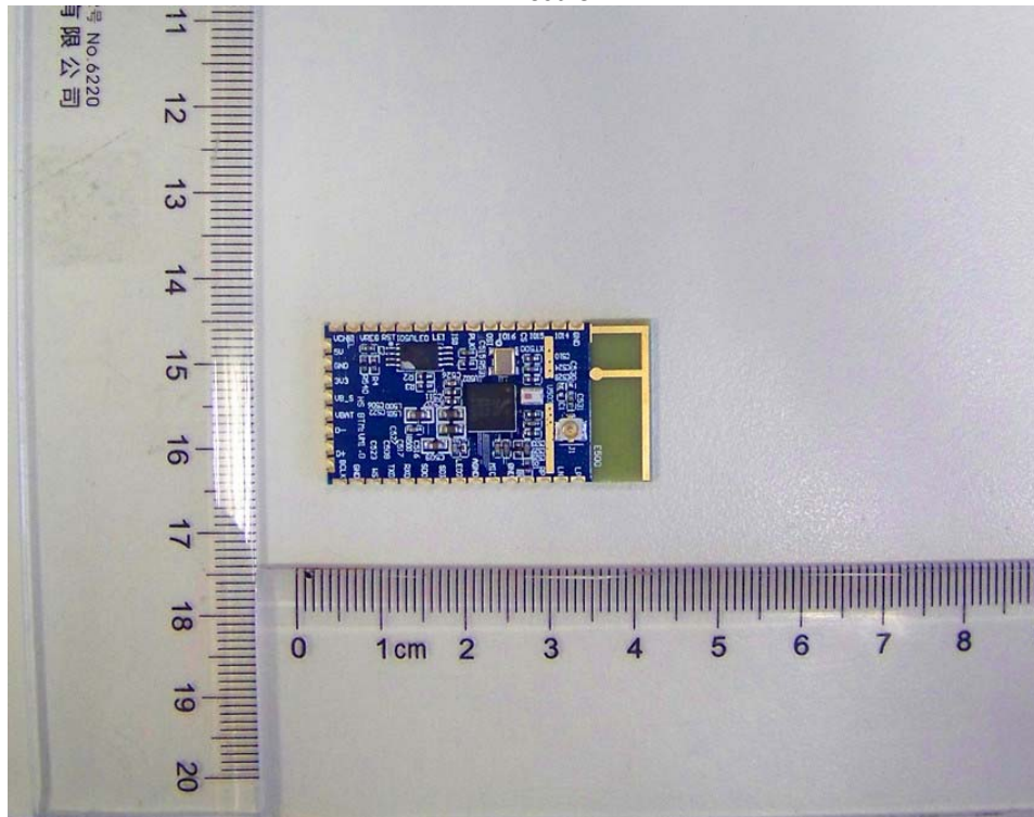
BT Module
