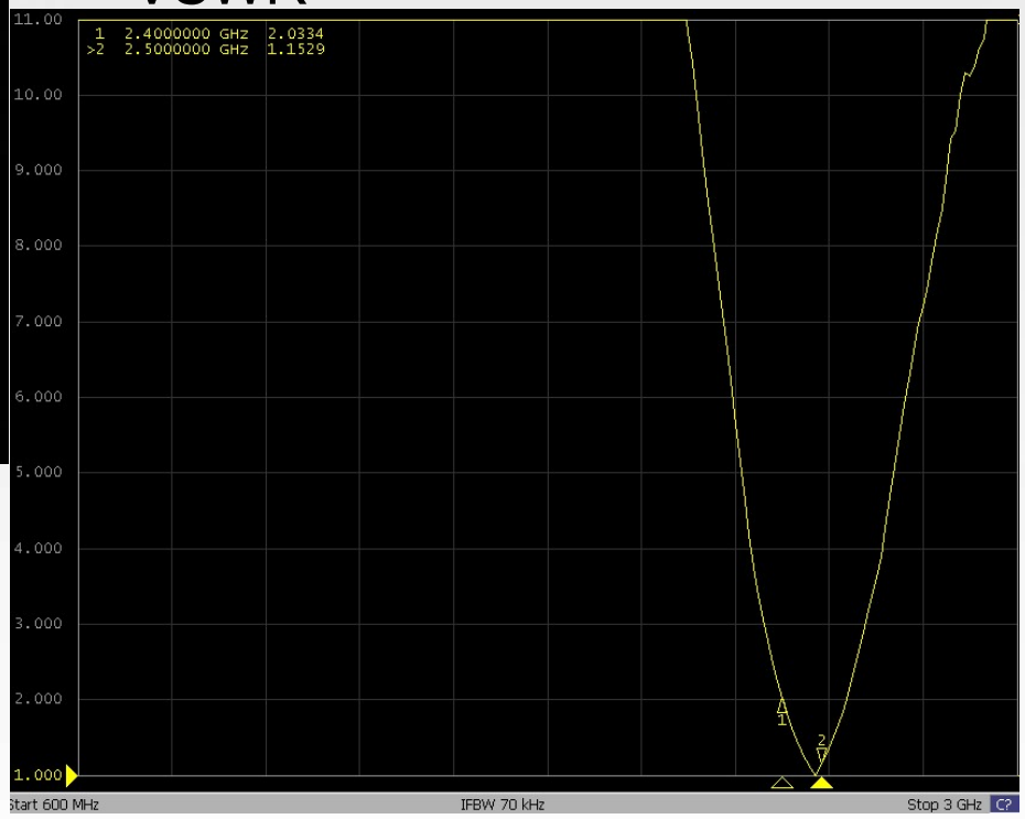
VSWR
