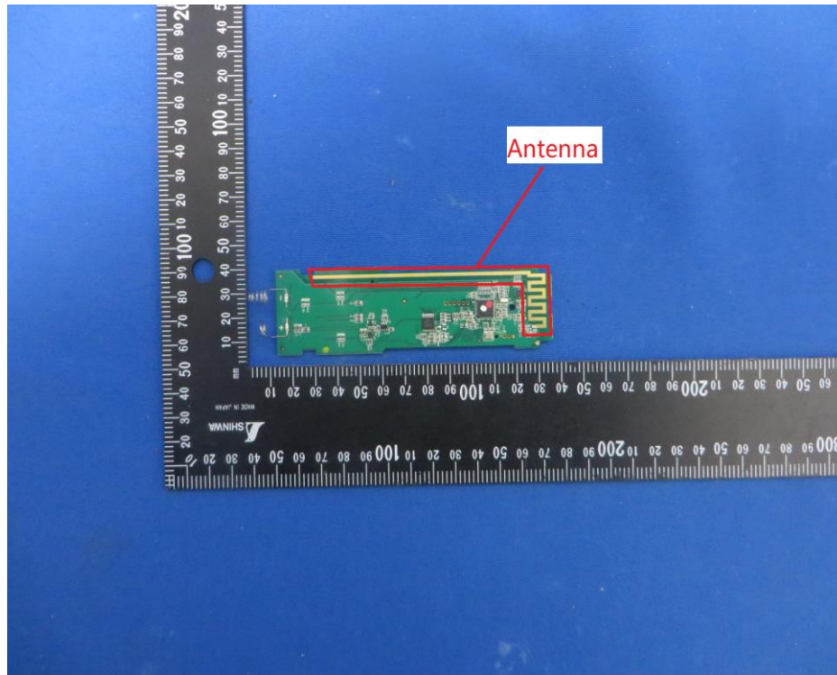
(3) EUT Photo
