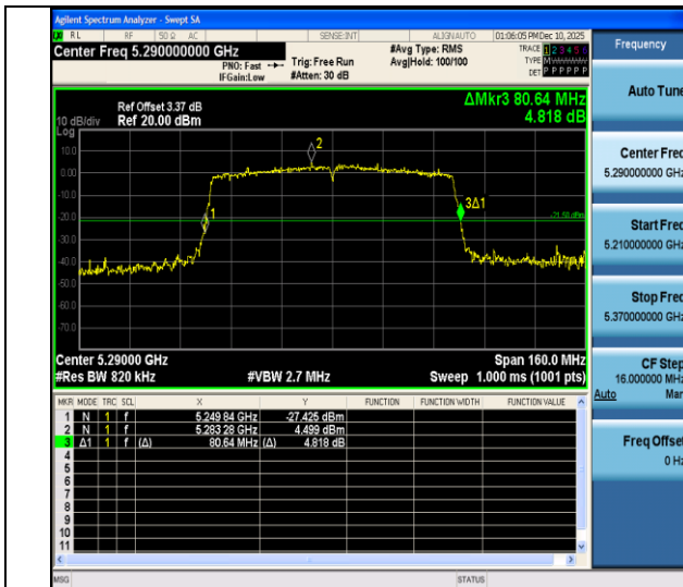
11ac80SISO-Ant4-5290
