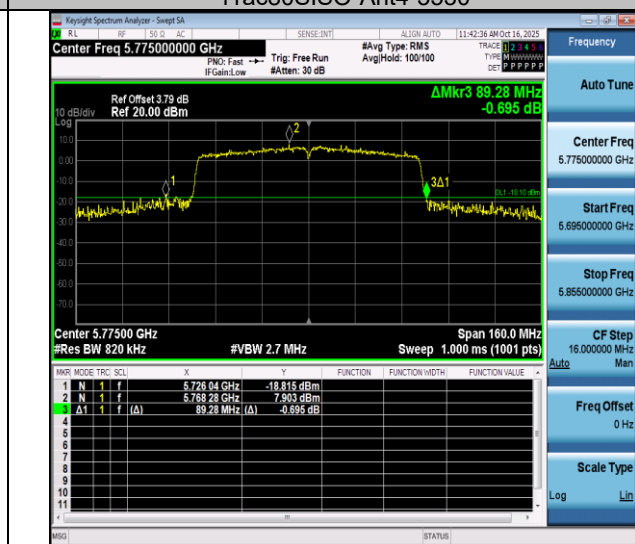
11ac80SISO-Ant4-5775
