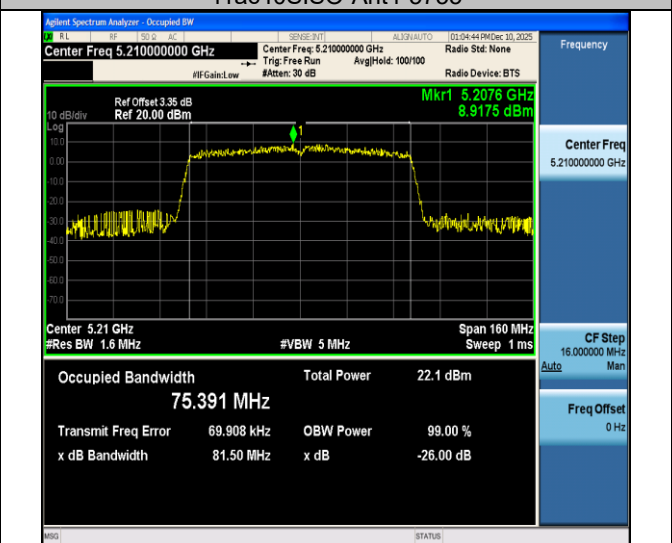
11ac80SISO-Ant4-5210
