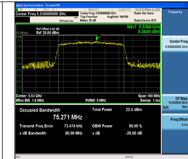
11ac80SISO-Ant4-5530
