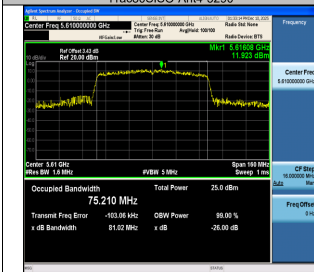
11ac80SISO-Ant4-5610
