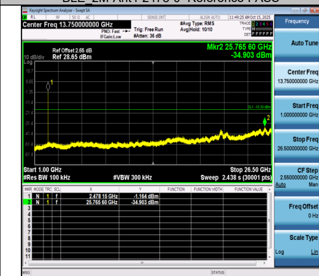
BLE 2M-Ant4-2478-1000~26500-PASS
