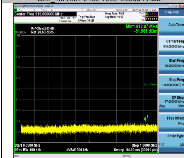
BLE 2M-Ant4-2404-30~1000-PASS
