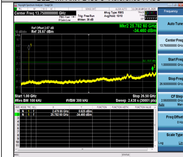
BLE 1M-Ant4-2480-1000~26500-PASS
