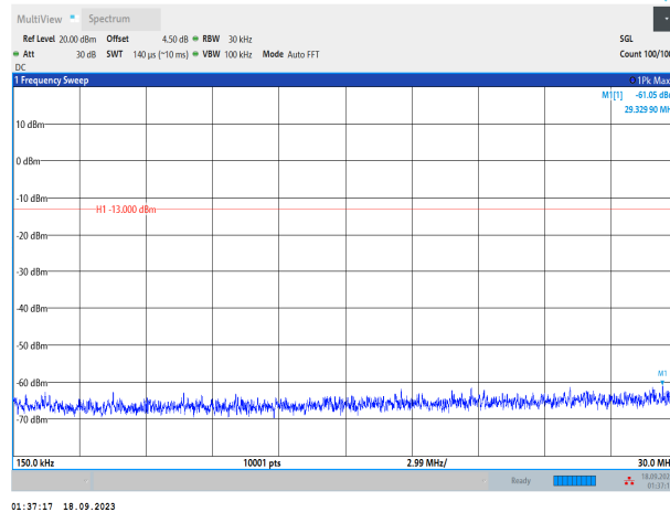
GSM850-128-0.15~30MHz
