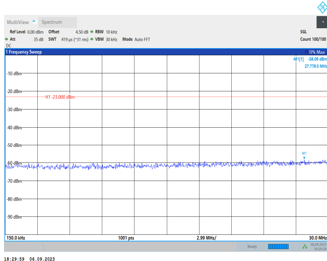
Band66-20MHz-QPSK-132072-1RB#0-Range2:0.15~30MHz
