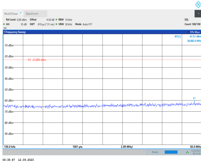
Band71-20MHz-QPSK-133222-1RB#0-Range2:0.15~30MHz
