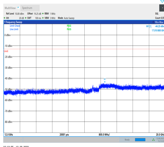
1-N71-PC3-15-20-M-1-DFT-PI2BPSK-Inner_1RB_Lef t-1@1-12000-20000-Ant1-17010.80--44.23--13-PASS
