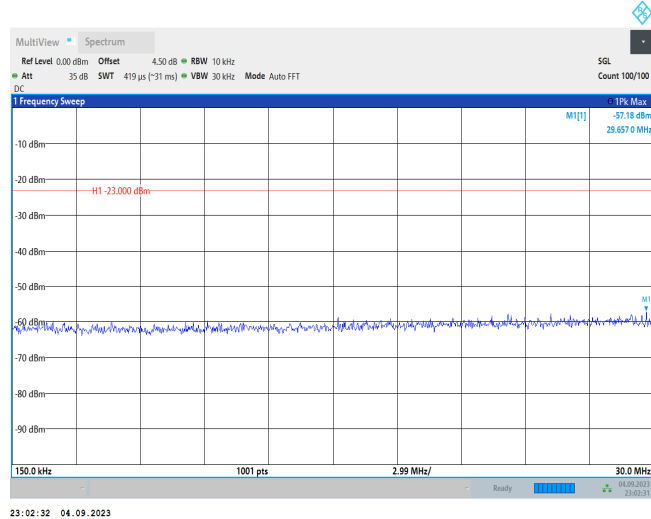
Band71-20MHz-QPSK-133222-1RB#0-Range2:0.15~30MHz
