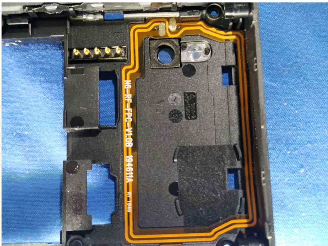
NFC Loop Antenna
