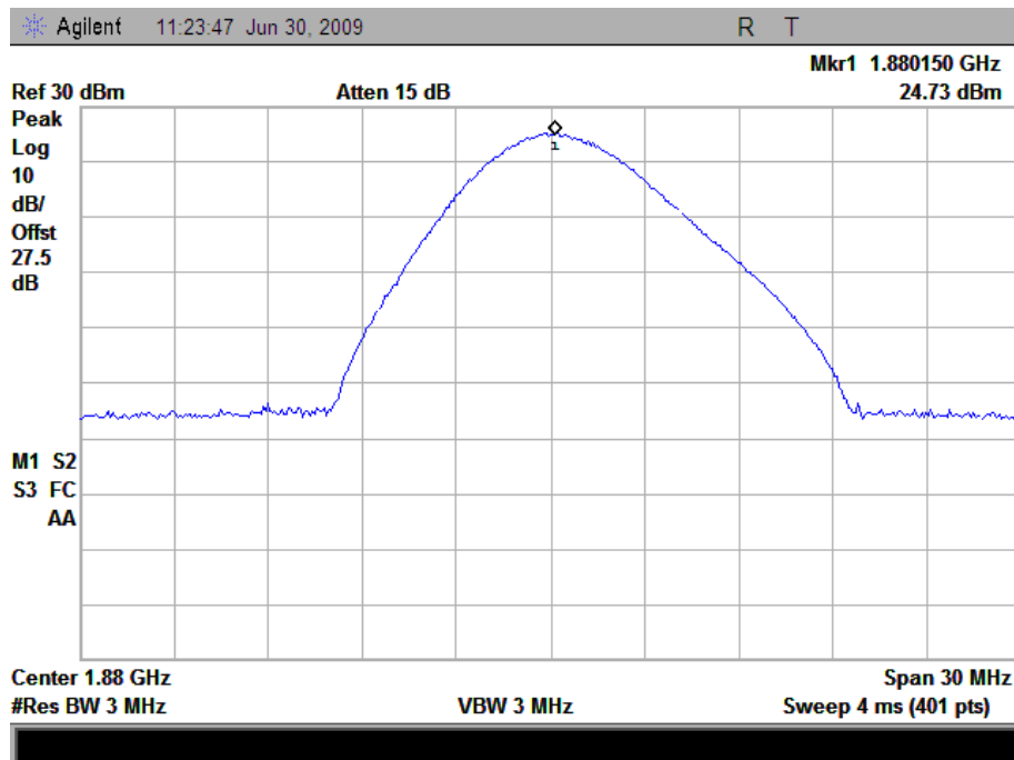
(Plot E: CDMA 1900MHz Channel = 600)
