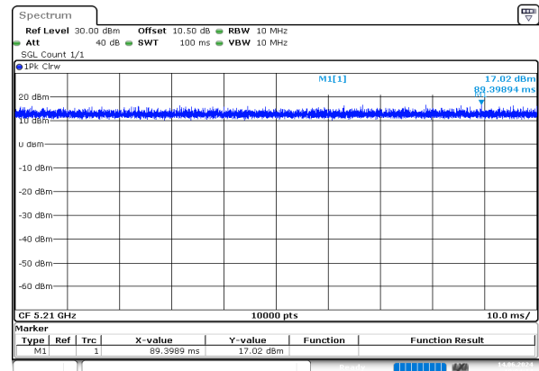
ac80_5210MHz_Chain 0
