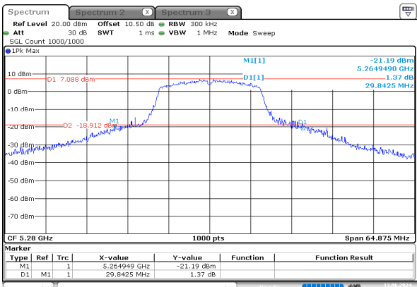
a_5280MHz_Chain 0
