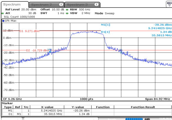
a_5260MHz_Chain 0
