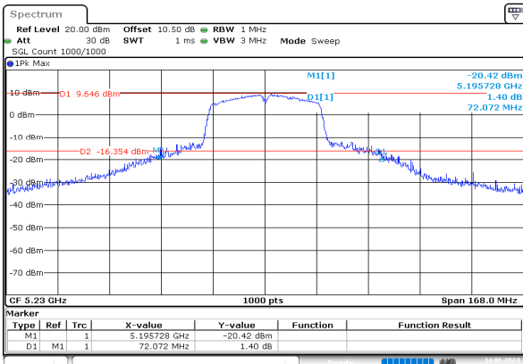
n40_5230MHz_Chain 0
