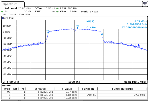
n40_5230MHz_Chain 0
