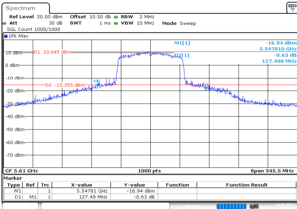
ac80_5610MHz_Chain 0
