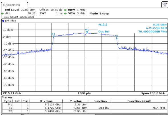
ac80_5210MHz_Chain
