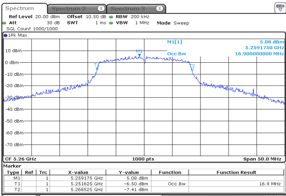
a_5260MHz_Chain 0
