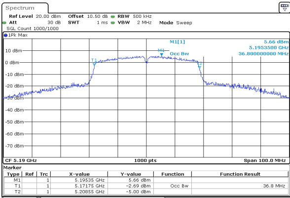
n40_5190MHz_Chain 0
