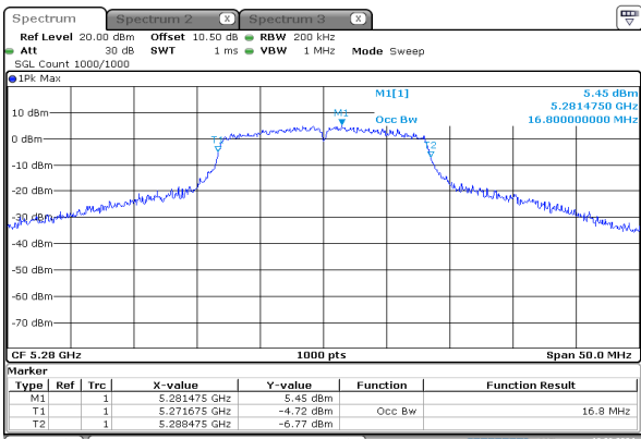
a_5280MHz_Chain 0
