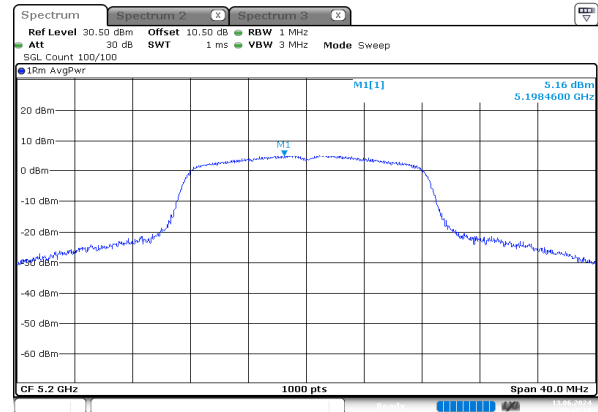
a_5200MHz_Chain 0
