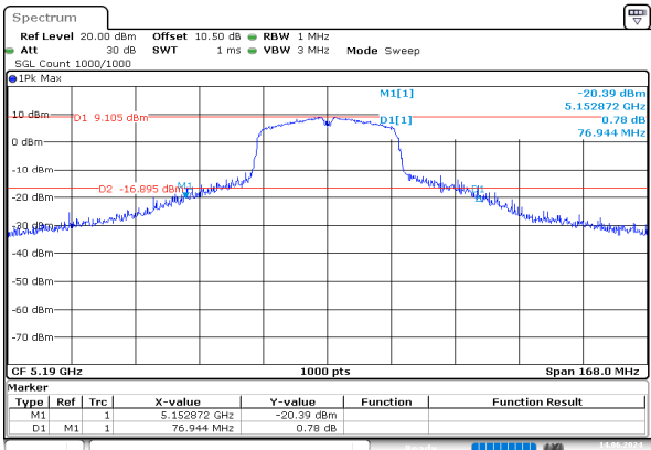
n40_5190MHz_Chain 0
