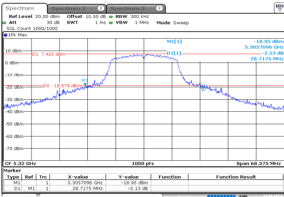
a_5320MHz_Chain 0
