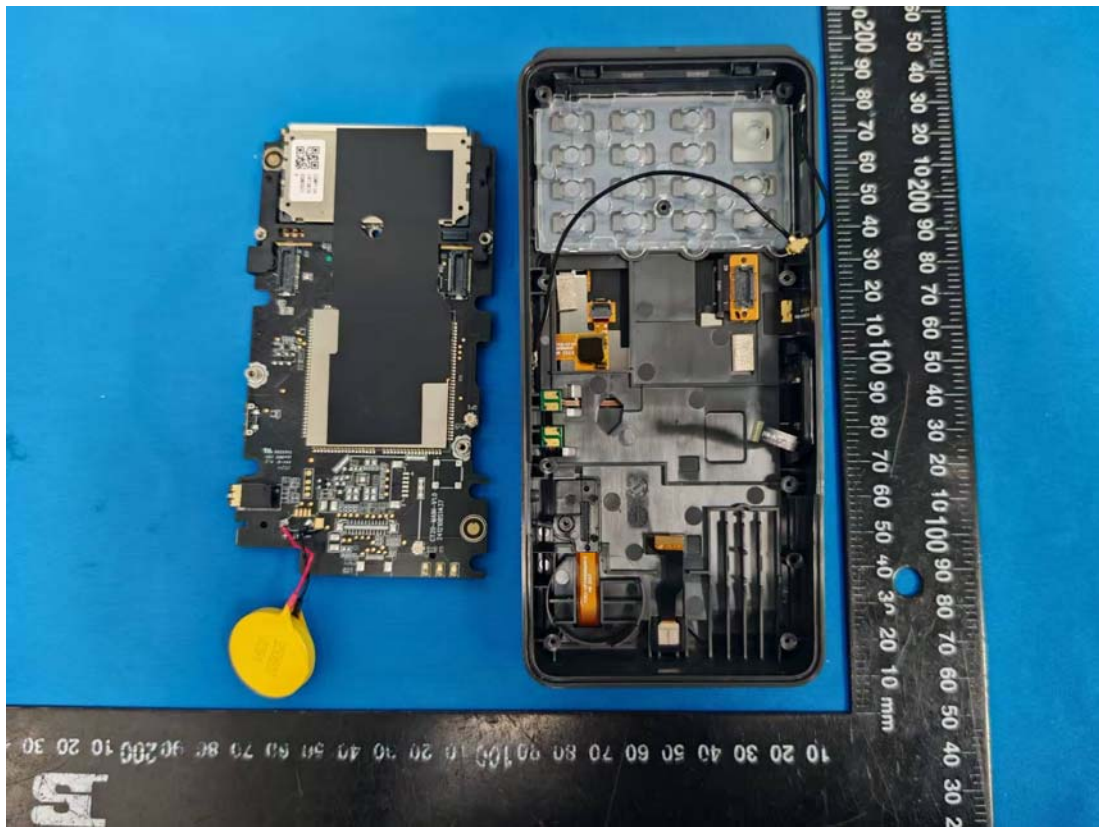
Bluetooth&Wifi Antenna
