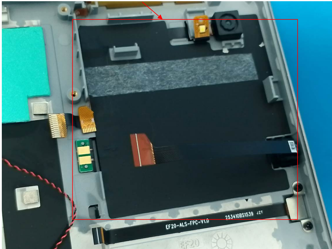
NFC Antenna(ANT 3)
