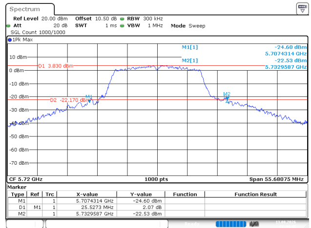
802.11a_5720MHz
