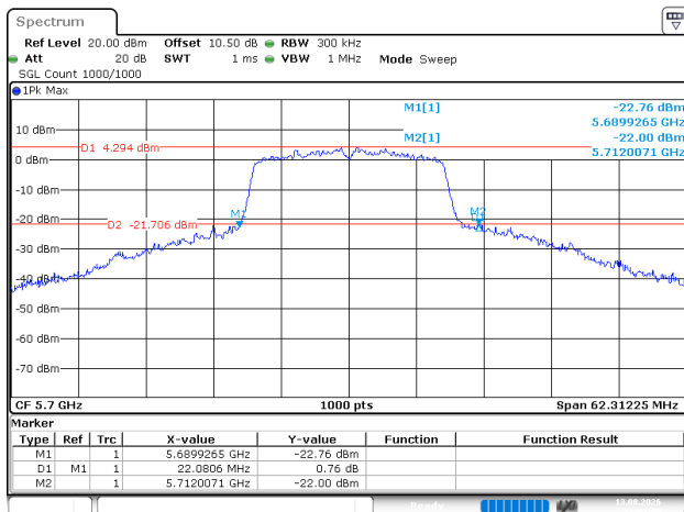
802.11n20_5700MHz
