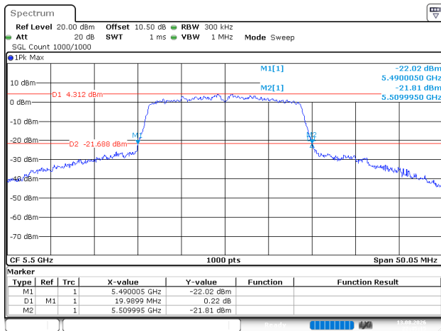
802.11n20_5500MHz
