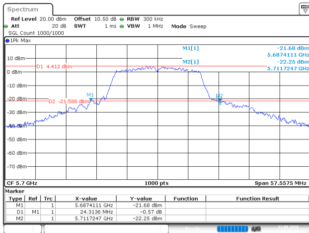
802.11a_5700MHz
