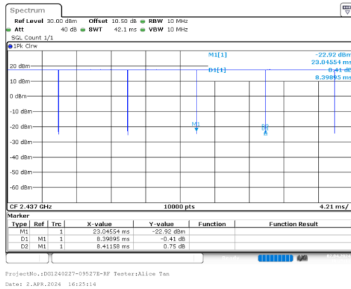
b_2437MHz_Chain 0
