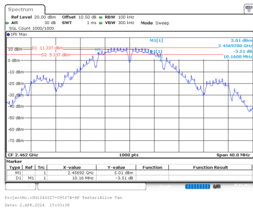
b_2462MHz_Chain 0
