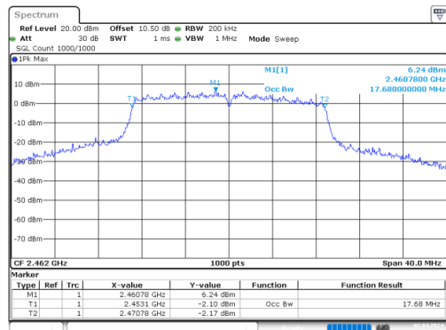
n20_2462MHz_Chain 0
