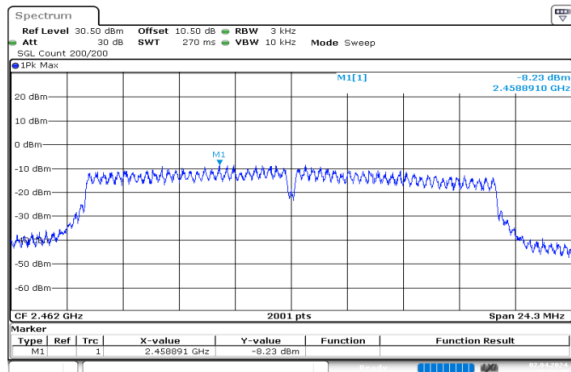
n20_2462MHz_Chain 0
