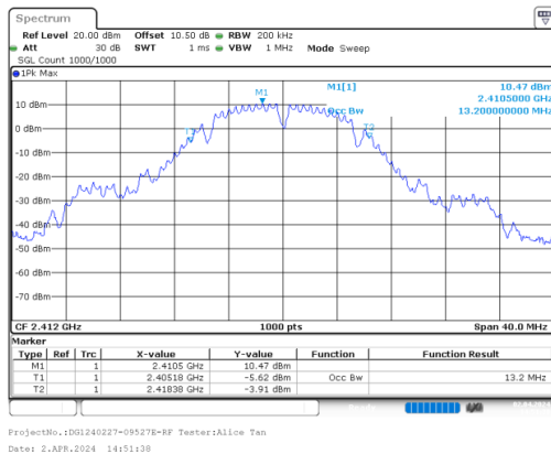
b_2412MHz_Chain 0
