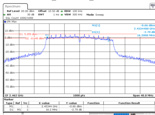
n20_2462MHz_Chain 0
