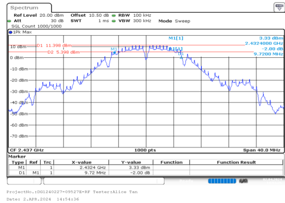
b_2437MHz_Chain 0
