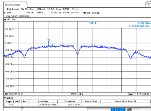
b_2462MHz_Chain 0
