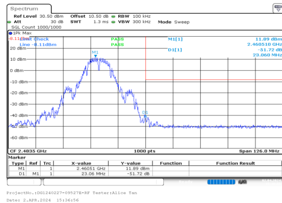
b_2462MHz_Chain 0
