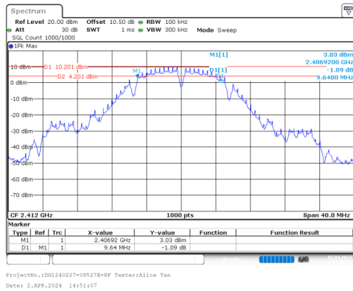
b_2412MHz_Chain 0
