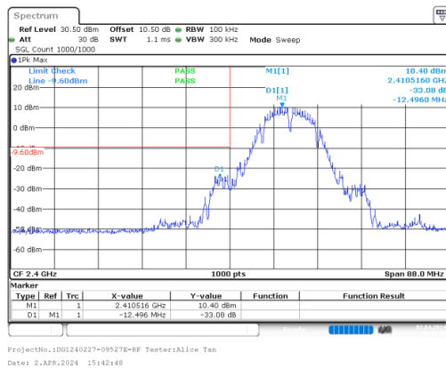
b_2412MHz_Chain 0
