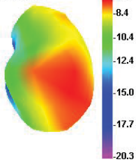
1720.000MHz
