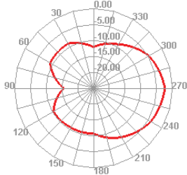
2700.000MHz E1
