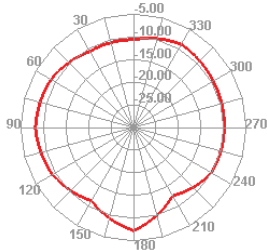
1720.000MHz E2
