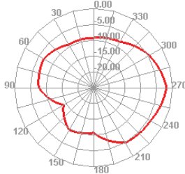
2700.000MHz E2
