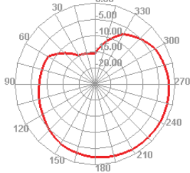
2700.000MHz H
