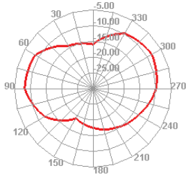
1720.000MHz H
