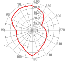
1720.000MHz E1
