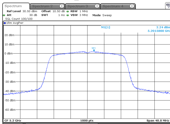
n20_5200MHz
