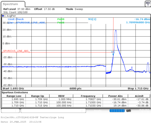
5MHz_Low_QPSK_1@0
