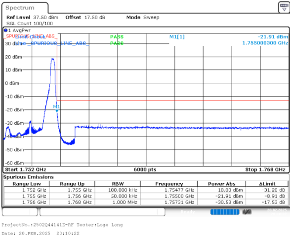
5MHz_Low_QPSK_1@0
