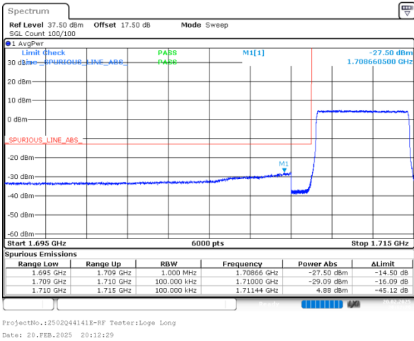
5MHz_Low_QPSK_25@0
