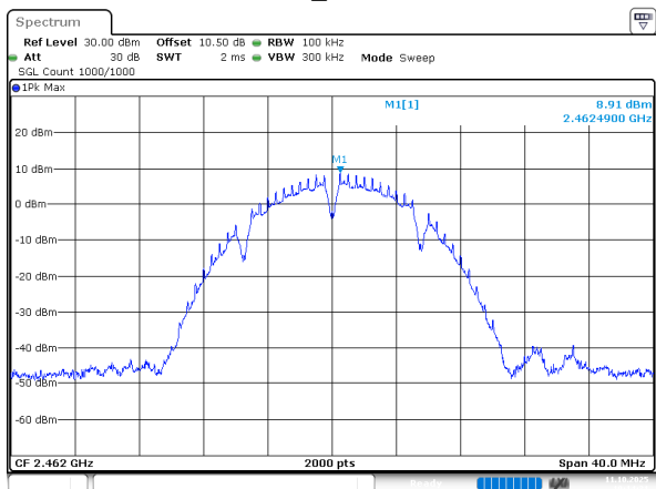
802.11b_2462MHz
