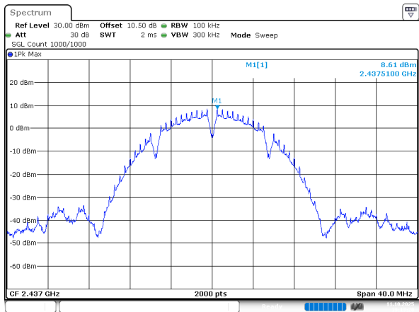
802.11b_2437MHz
