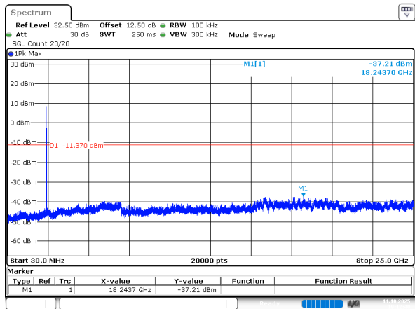
802.11b_2412MHz
