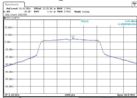
n20_5180MHz
