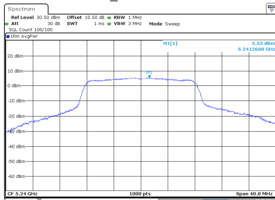
a_5240MHz
