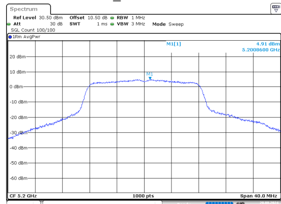
a_5200MHz
