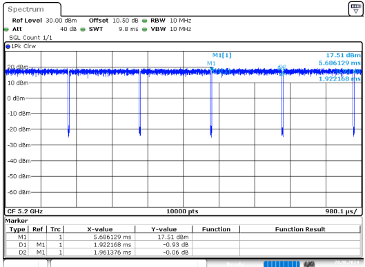
n20_5200MHz
