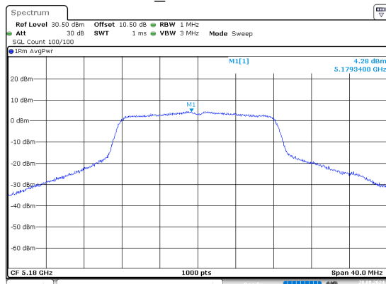
a_5180MHz
