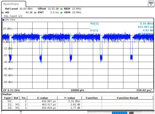
ac80_5210MHz
