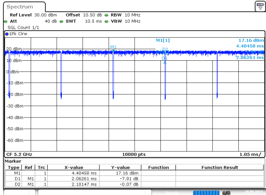
a_5200MHz
