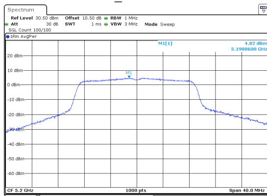
n20_5200MHz
