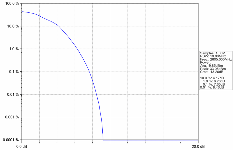
Band41_10MHz_16QAM_MCH_2605MHz_RB_50_0_NTNV
