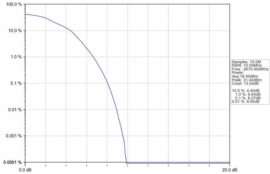
Band41_10MHz_16QAM_HCH_2670MHz_RB_50_0_NTNV
