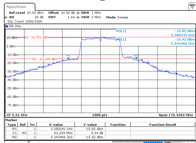
802.11ac40_5310MHz
