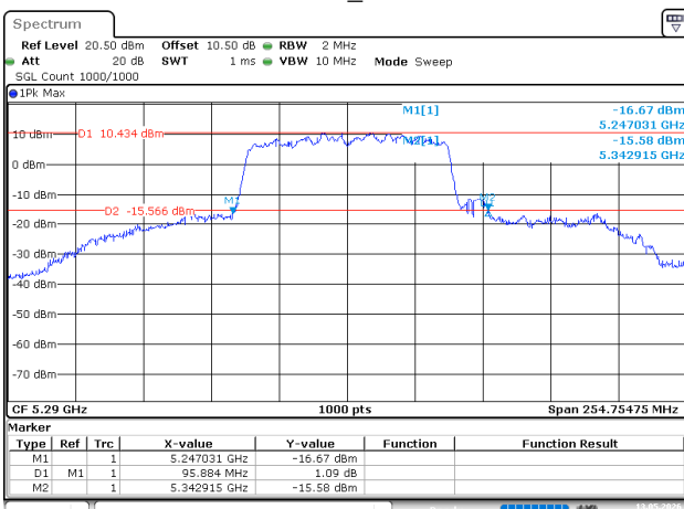
802.11ac80_5290MHz
