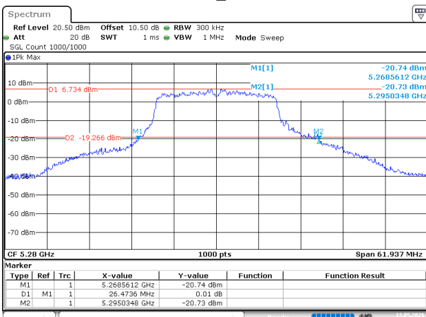
802.11ac20_5280MHz
