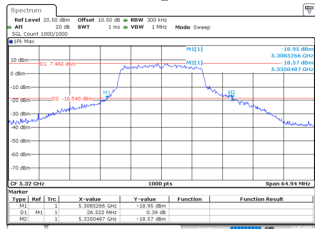
802.11ac20_5320MHz
