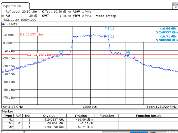
802.11ac40_5270MHz
