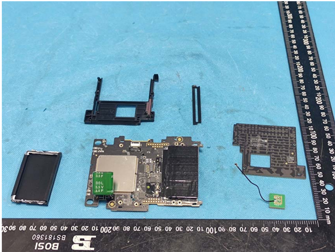
GPS Antenna
