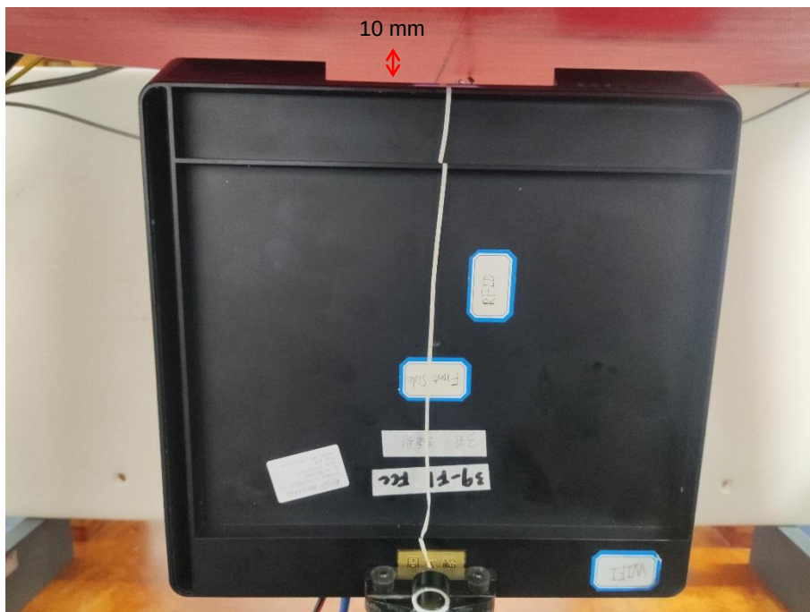
Bottom Edge (10mm)-RFID
