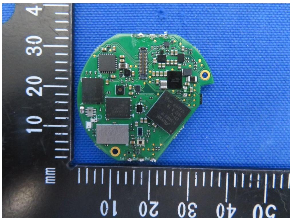
(10) EUT Photo
