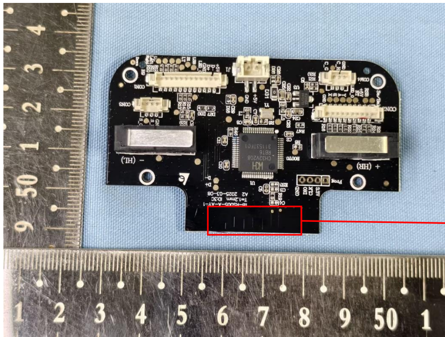
2.4G Antenna
