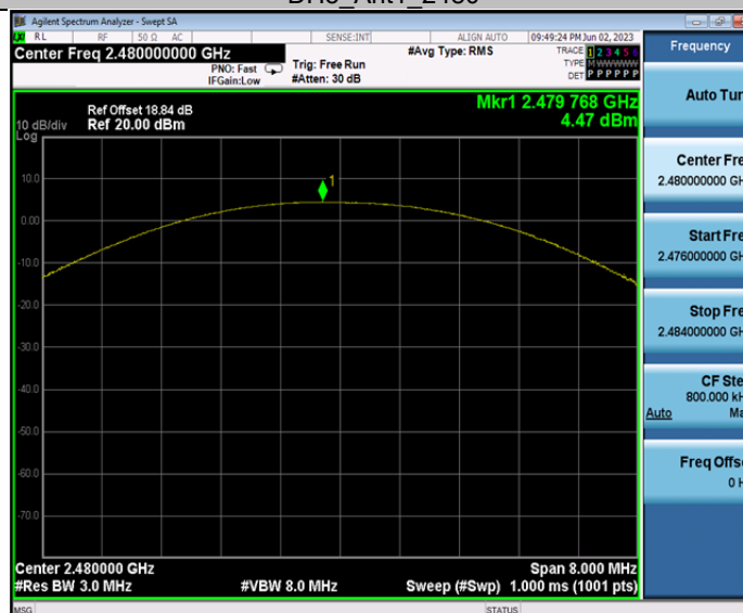
DH5_Ant1_2480
